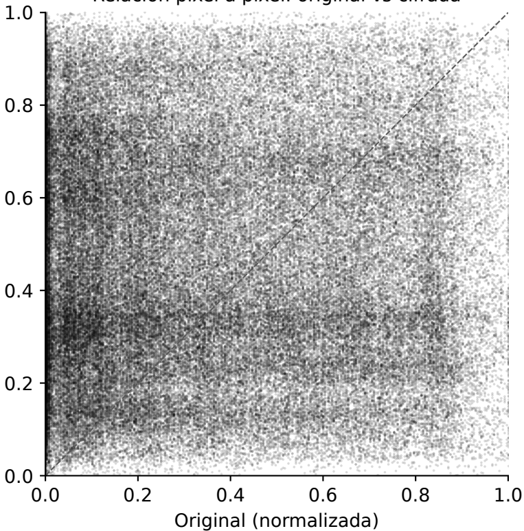
Relación píxel a píxel: original vs cifrada
