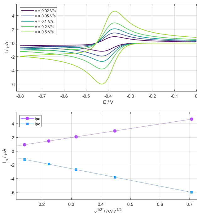
Figure 1 — Couple rapide ( k^0 = 1 \text{ cm}^2/\text{s} ), cinq vitesses de 0,02 à 0,5 V/s : voltammogrammes et droites I_p = f(v^{1/2}) calculées par la fenêtre Series.
