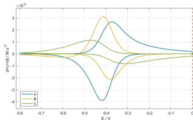
Figure 2 — Couche stagnante de 200 \mu\text{m} , A + e = B suivi de B \rightarrow C ( k = 0,05 \text{ s}^{-1} ), 10 mV/s : dérivée de la concentration moyenne de A, B et C sur la couche.
