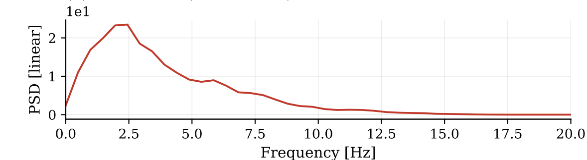
(b) Welch PSD (linear scale)
