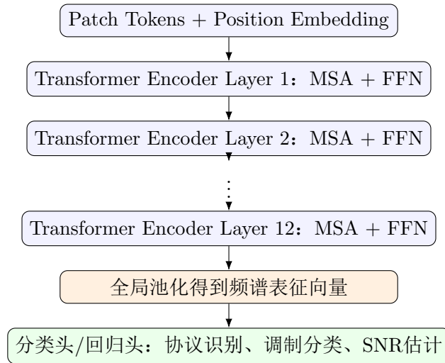
图 9 LWM-Spectro编码器结构示意图
