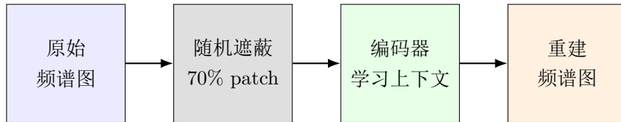
图 7 掩码频谱建模（MSM）自监督预训练示意
