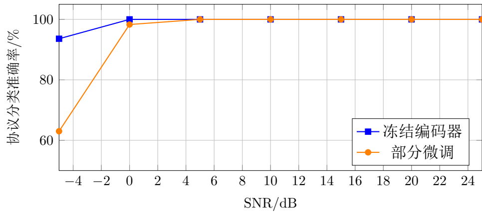
图 8 不同 SNR 条件下协议分类准确率示意（根据技术报告结果重绘）
