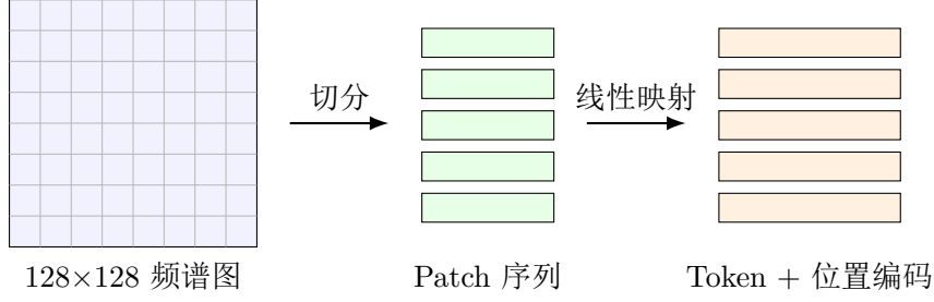
图 5 频谱图 Patch Embedding 原理示意
