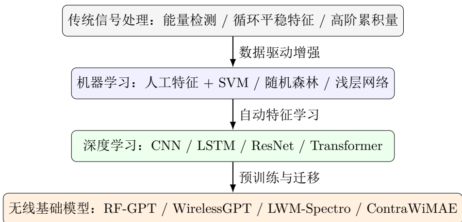
图 3 频谱认知技术的演进路线
