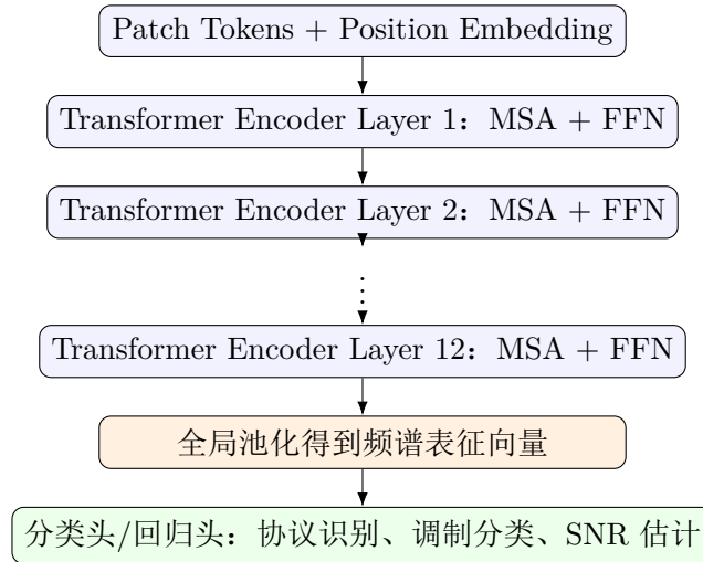
图 6 LWM-Spectro 编码器结构示意图
