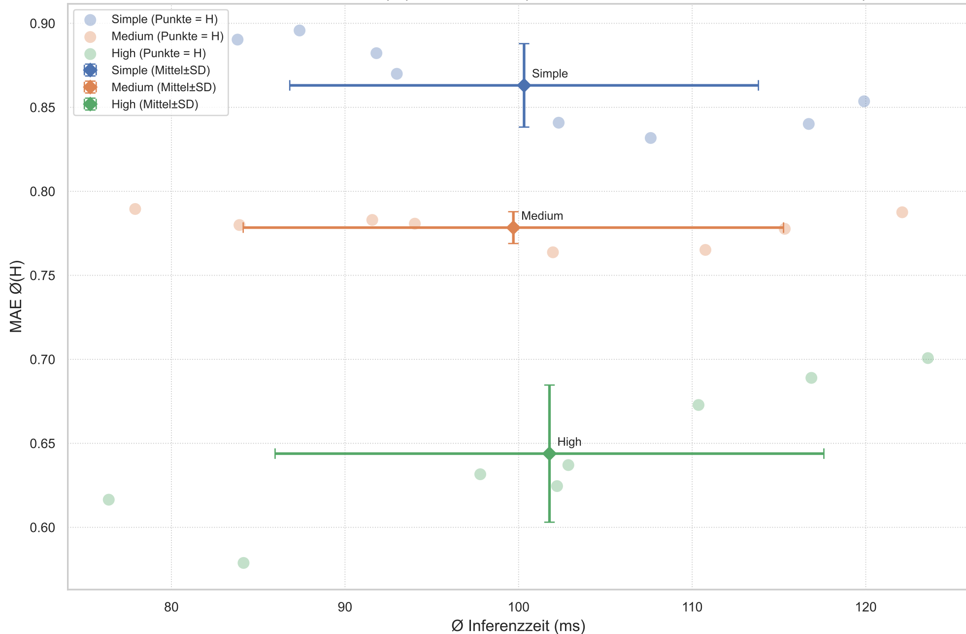
Inferenzzeit vs. MAE \emptyset(H) über Level (H als Punkte, Level-Mittel als Raute)
