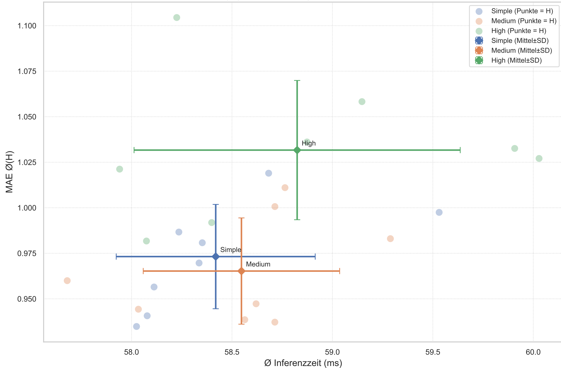
Istm — no-quant Inferenzzeit vs. MAE \emptyset(H) über Level (H als Punkte, Level-Mittel als Raute)
