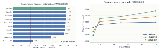
Figure 1: 第二轮频域优化和抽样比例扩大带来的 clean performance 提升。
