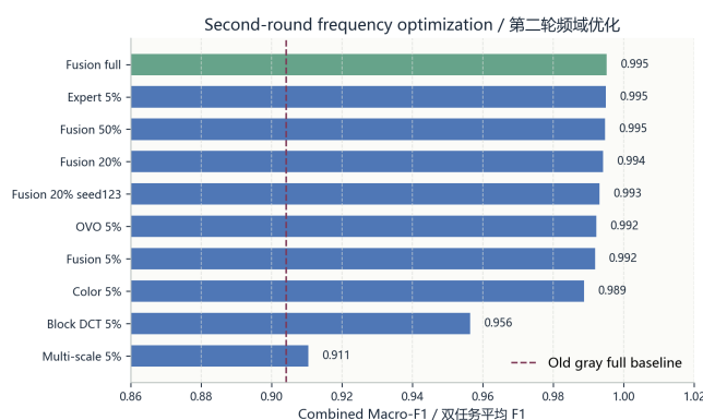
Figure 1: 第二轮频域优化和抽样比例扩大带来的 clean performance 提升。
