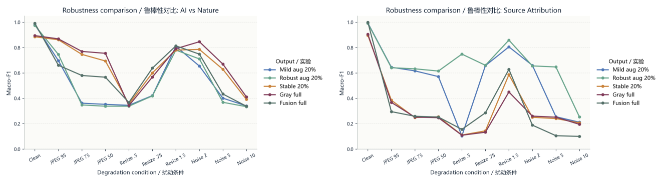
Figure 9: 当前 fusion_freq 最佳模型与旧灰度 baseline 的 degraded validation 对照。
