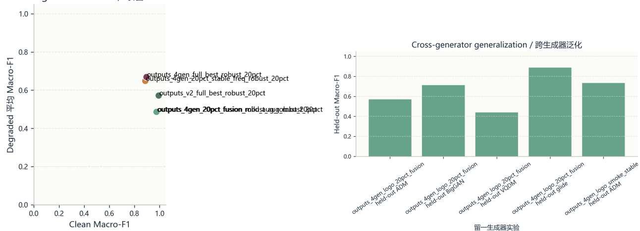
Figure 10: 左: clean 与 degraded 平均 F1 的取舍; 右: leave-one-generator-out 泛化结果。
