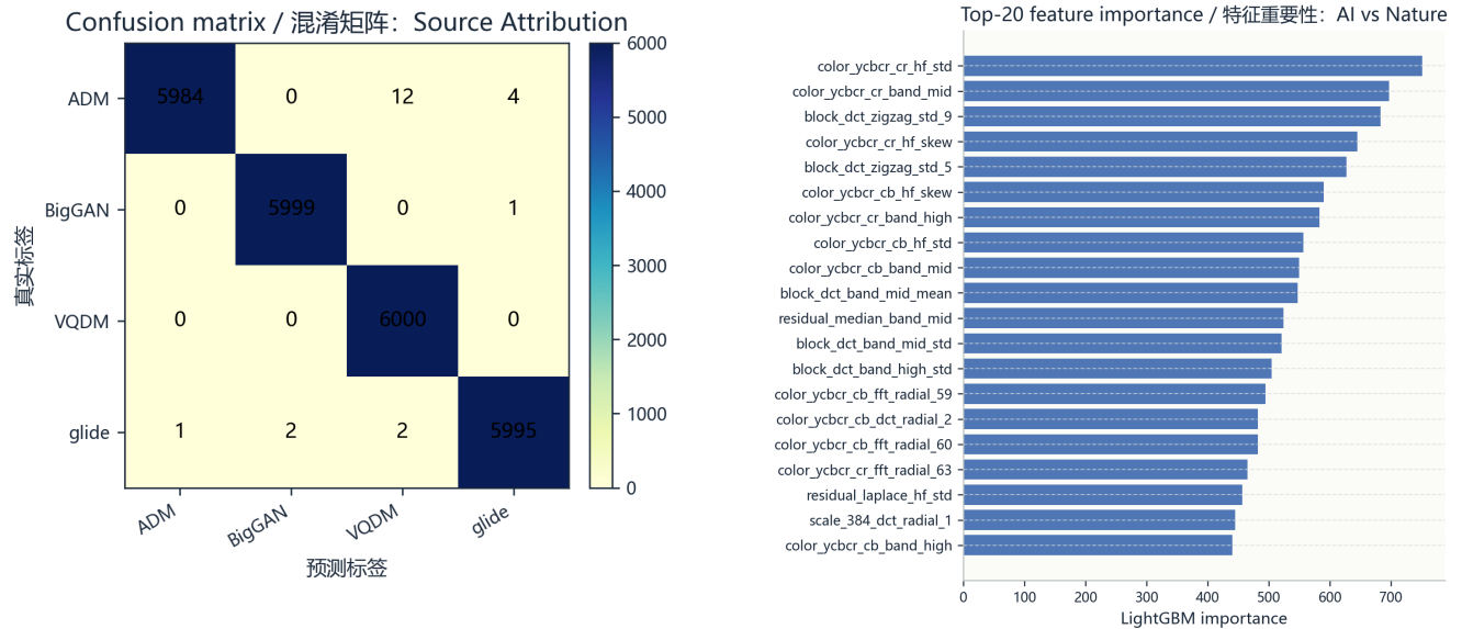
Figure 7: 最终 full 模型在生成源归因任务上的混淆矩阵。
