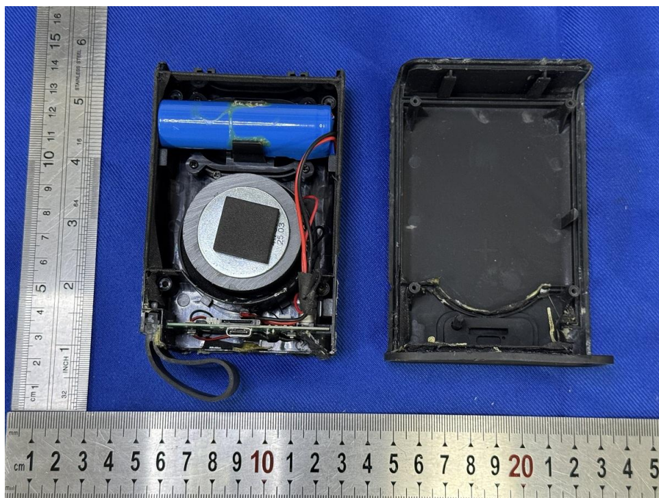
图四 IP6X 测试后
