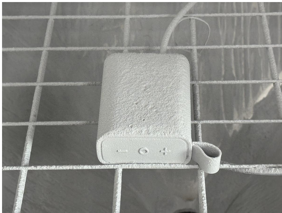
图三 IP6X 测试中
