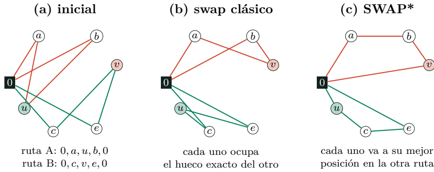
Figura 3: Diferencia entre el swap clásico y SWAP*. Los puntos no se mueven; solo cambian las rutas. En (a), u está mal ubicado en la ruta roja y v en la verde. El swap clásico (b) los intercambia, pero cada uno queda en el hueco que dejó el otro, lejos de donde conviene. SWAP* (c) los intercambia y coloca a cada uno en su mejor posición, así que encuentra mejoras que el swap clásico descarta.
