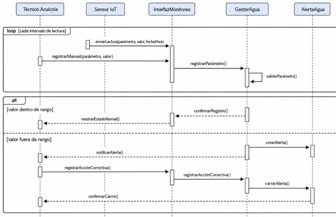
Figura 16: Diagrama de Secuencia: caso de uso CU-02 registrar parámetros del agua.
