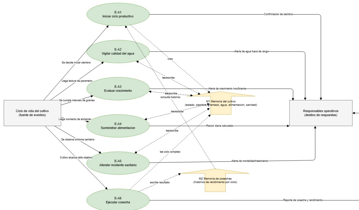
Figura 13: DFD Esencial: diagrama esencial del proceso principal del sistema AquaGest.
