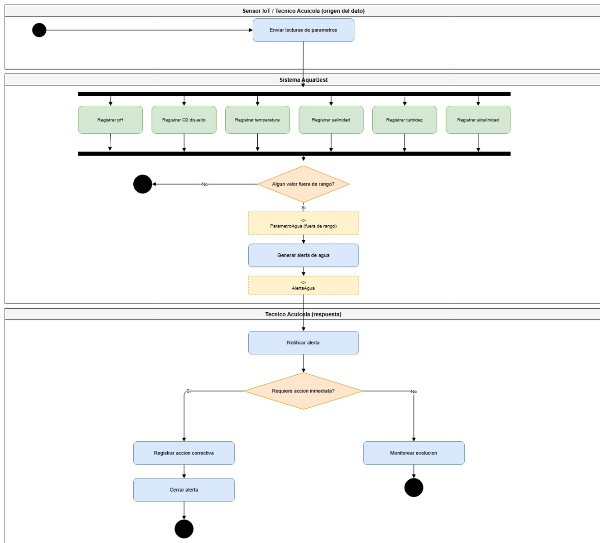
Figura 14: Diagrama de Actividades: diagrama de actividades del caso de uso principal del sistema AquaGest.
