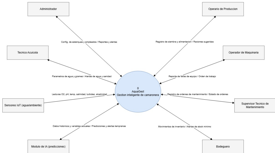
Figura 11: DFD Nivel 0: diagrama de contexto del sistema AquaGest.
