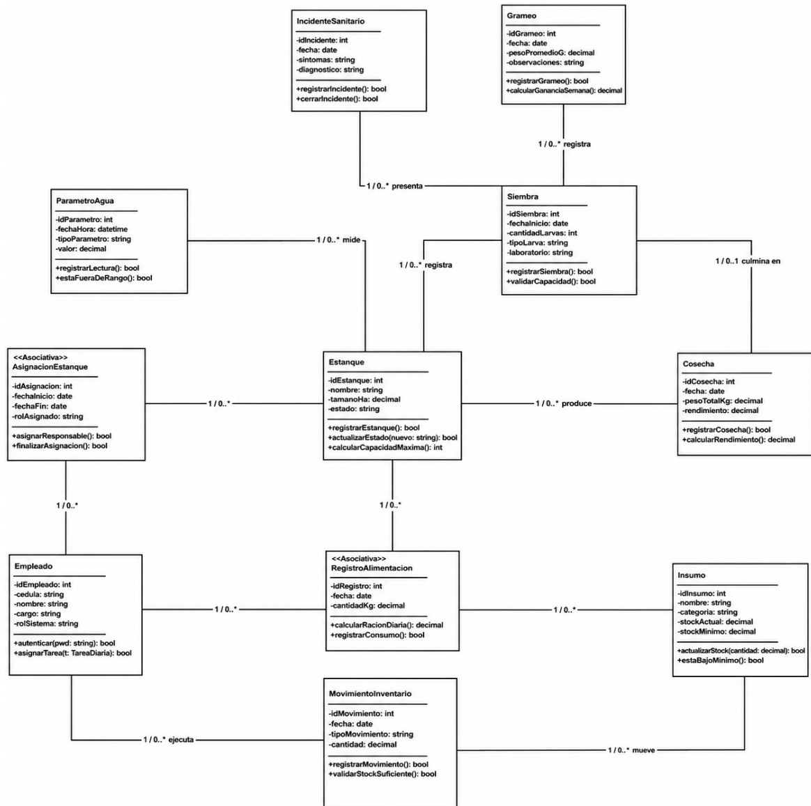
Figura 10: Diagrama de Clases UML del sistema AquaGest.
