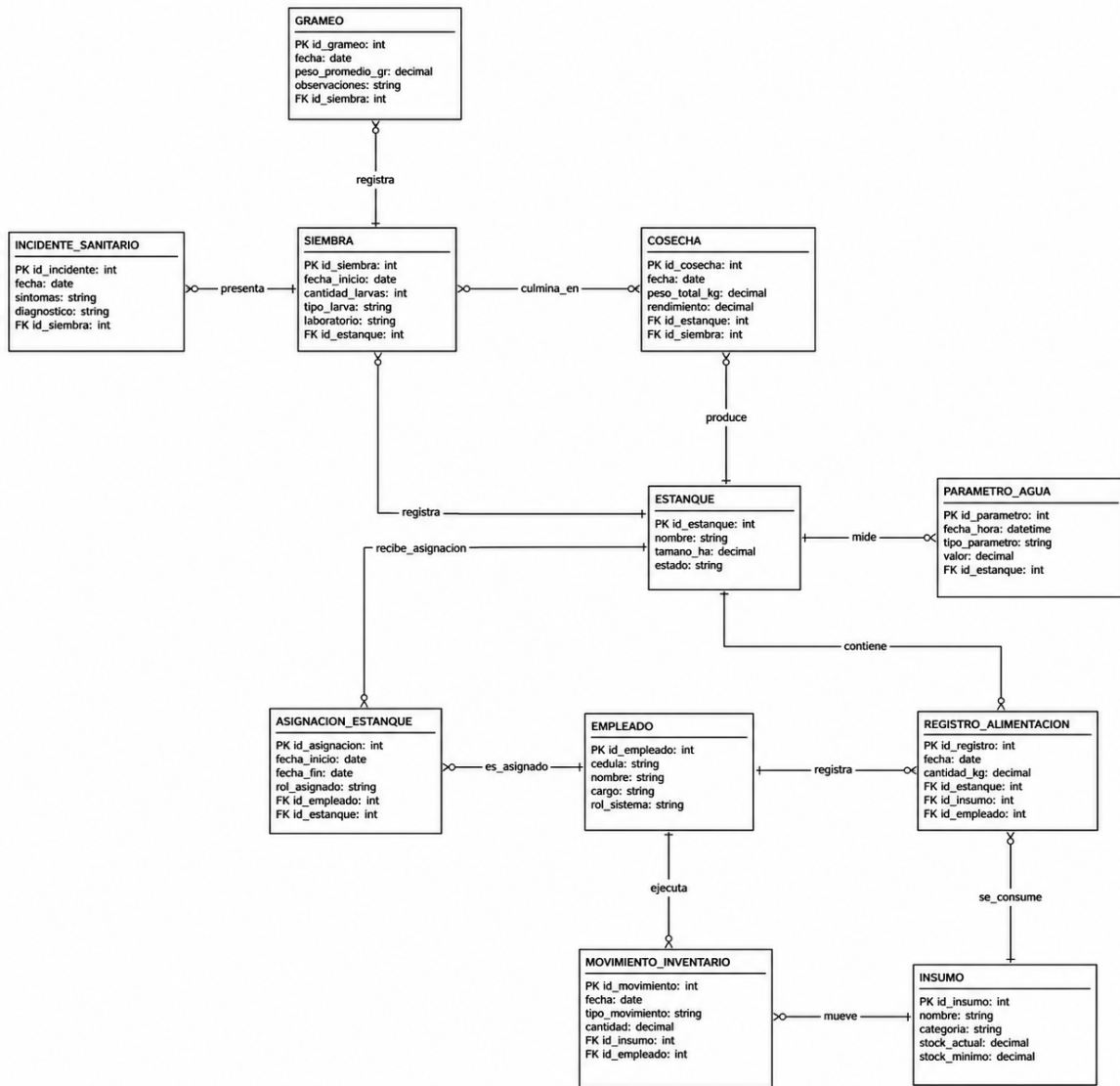
Figura 9: Diagrama ER del sistema AquaGest en notación Crow's Foot.
