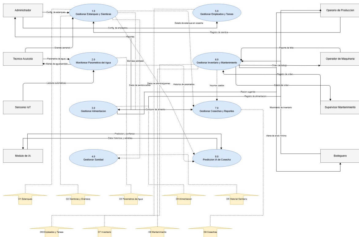
Figura 12: DFD Nivel 1: diagrama de nivel 1 del sistema AquaGest.
