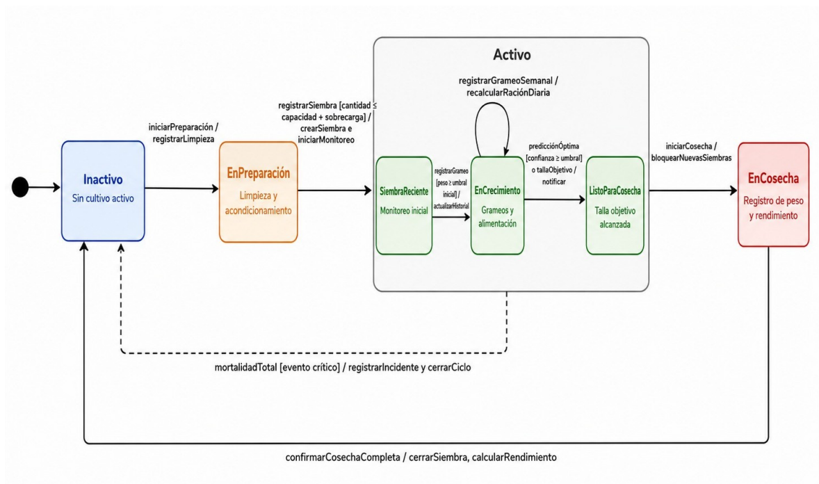
Figura 15: Diagrama de Máquina de Estados del sistema AquaGest.
