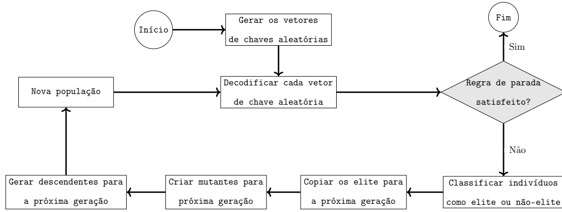
Figura 3: Fluxograma passo-a-passo do BRKGA.
