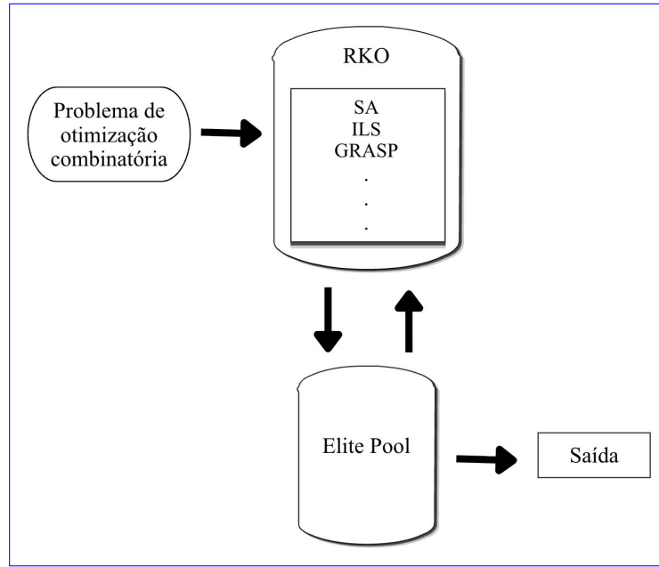
Figura 4: Fluxo geral do RKO.
