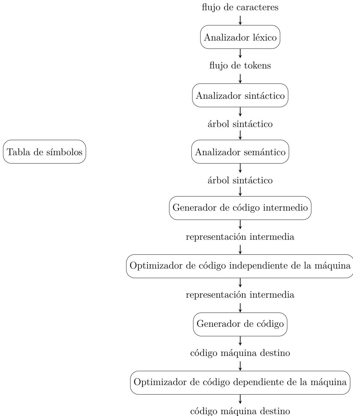
Figura 2.5: Fases de un compilador [3].
