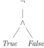
Figura 2.7: Árbol de sintaxis abstracta para (\neg(True \wedge False)) .
