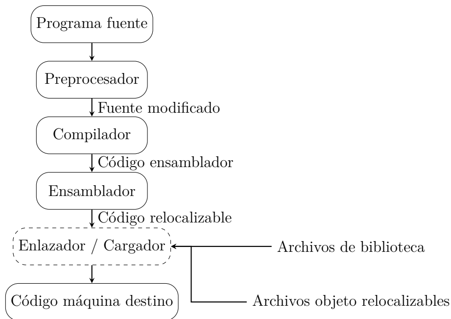
Figura 2.4: Un sistema de procesamiento de lenguaje [3].
