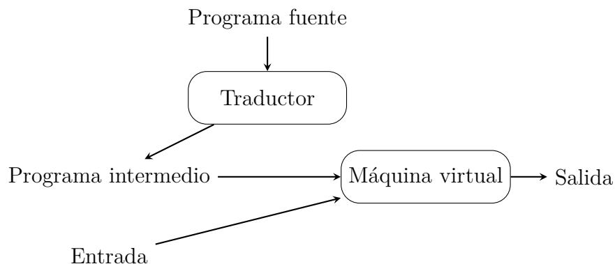
Figura 2.3: Combinación de compilación e interpretación [3].
