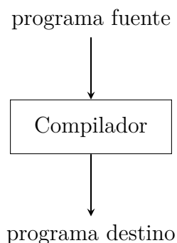
Figura 2.1: Un compilador [3].
