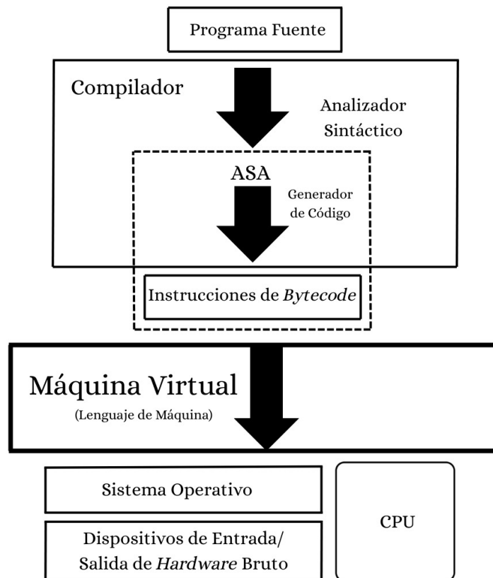
Figura 2.9: Implementación de una máquina virtual[45].
