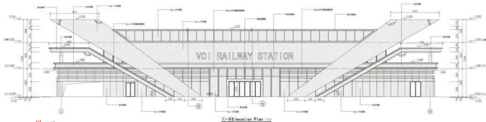
Elevation
