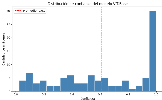
Figure 1: Distribución de confianza del modelo ViT-Base aplicado al dataset Caltech-101.
