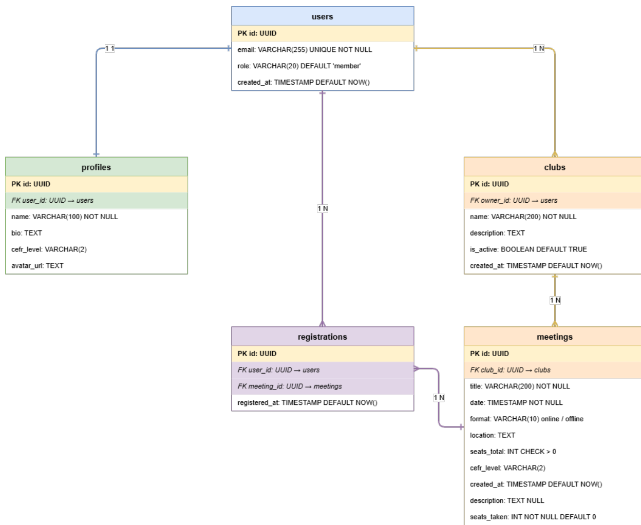
Рисунок 2.2 – ER-диаграмма базы данных
