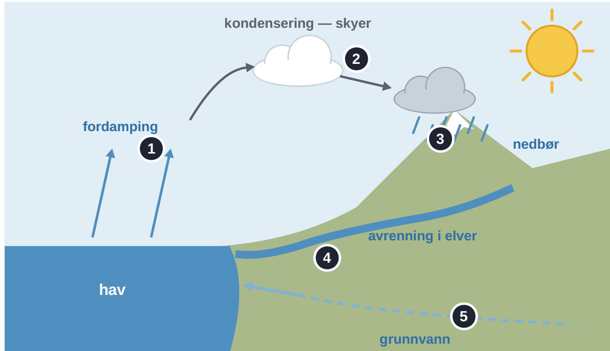
Figur 1.12 Vannets kretsløp.
