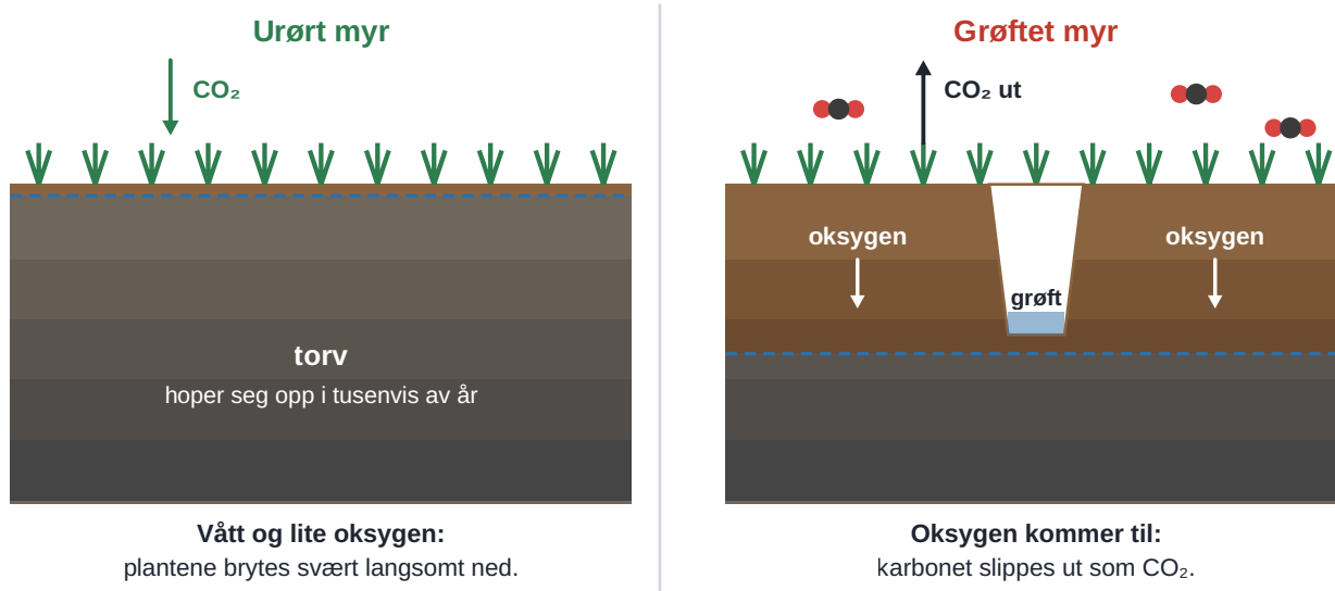
Figur 5.25 Urørt myr lagrer karbon. Grøftet myr slipper karbonet ut som CO 2 .
