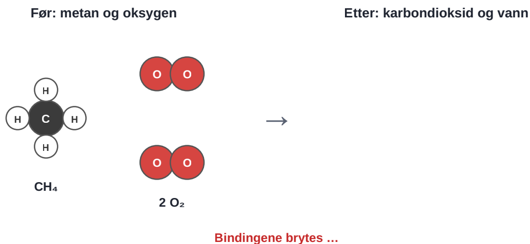
Figur 5.14 Metan brenner: atomene i \text{CH}_4 og \text{O}_2 blir satt sammen til \text{CO}_2 og \text{H}_2\text{O} .
