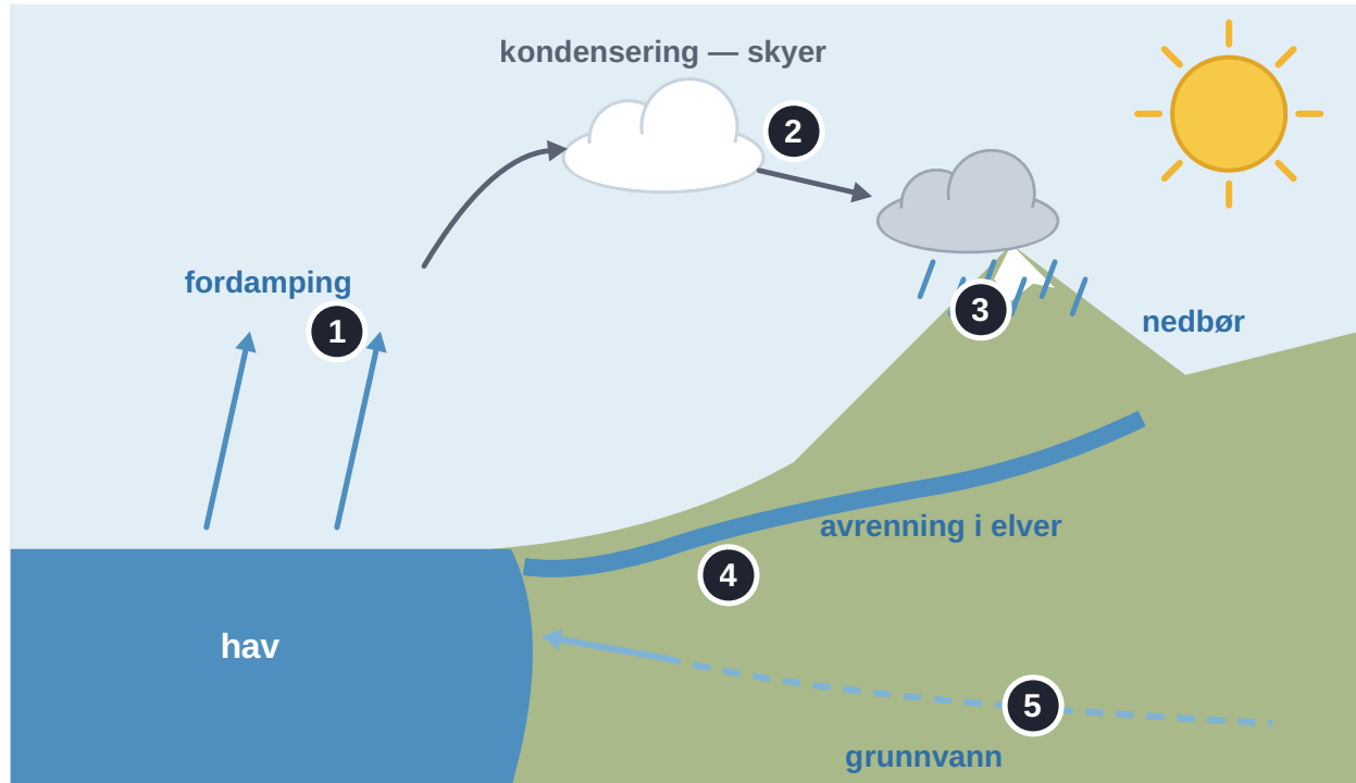
Figur 1.12 Vannets kretslop.
