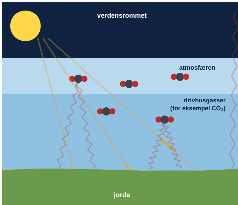
Figur 7.17 Drivhuseffekten: sollys inn, varmestråling ut, og noe av varmen sendes tilbake.
