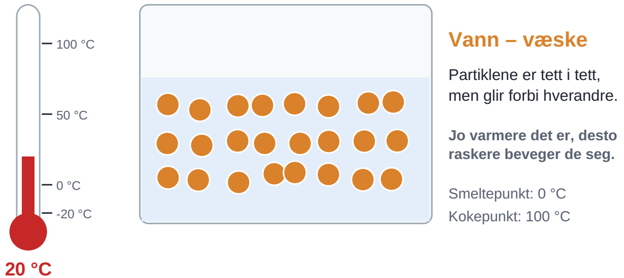
Figur 5.1 Prøv selv: vann som is, væske og damp. På nettsiden kan du endre temperaturen.
