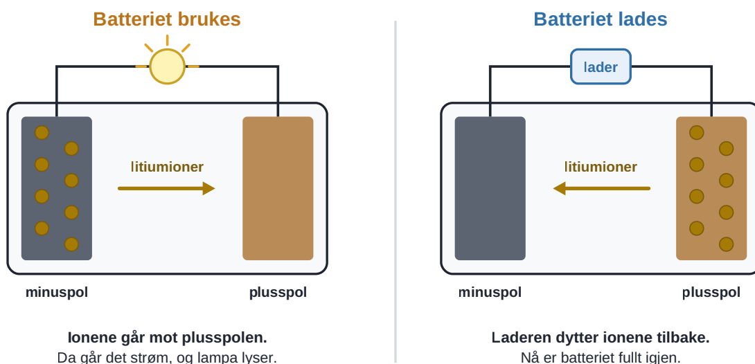
Figur 7.35 Et litium-ion-batteri som brukes og lades.
