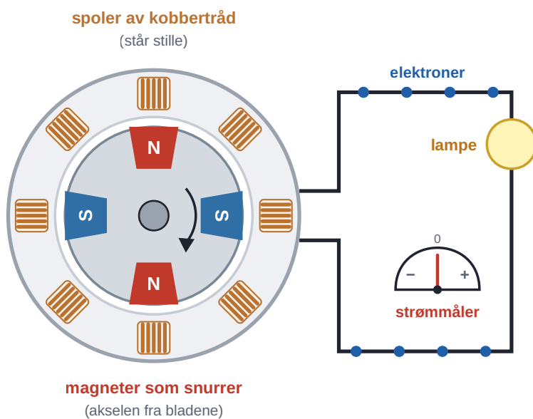
Figur 7.30 Inne i generatoren: magneter snurrer forbi spoler av kobbertråd, og elektronene blir dyttet fram og tilbake (vekselstrøm).
