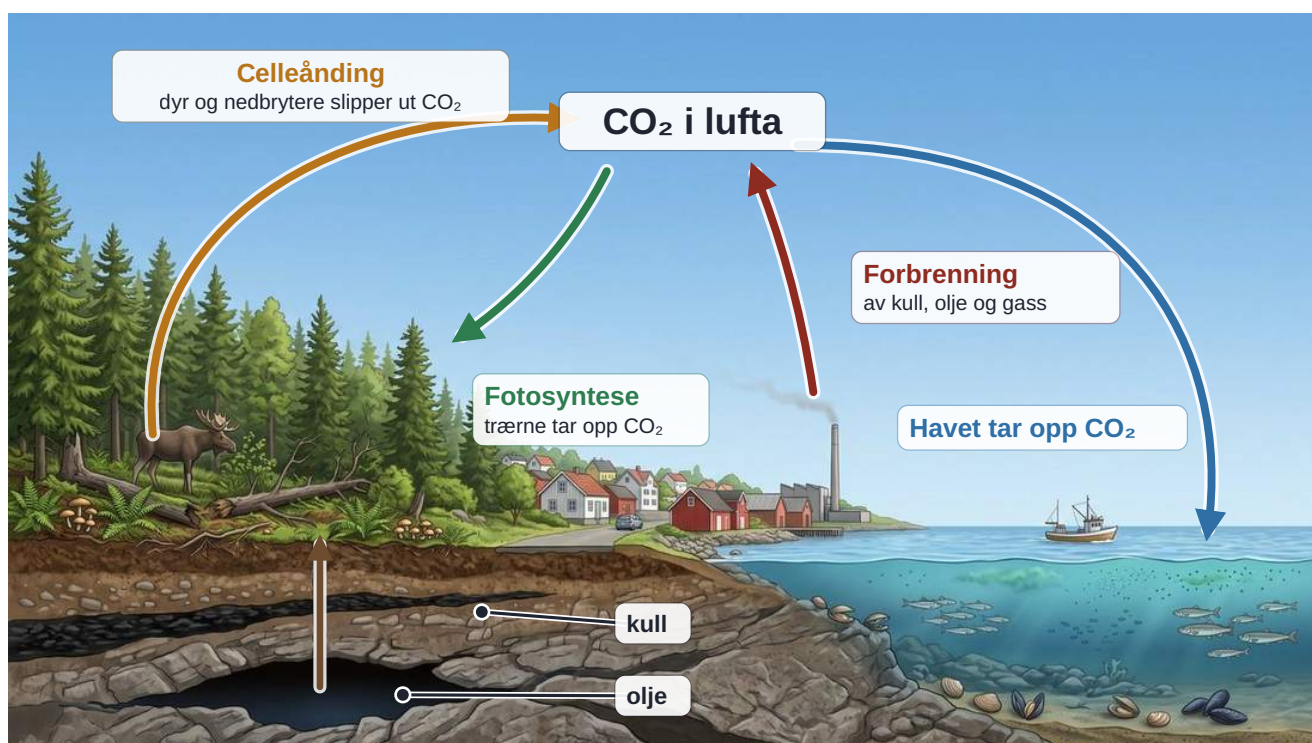
Figur 5.26 Karbonets kretsløp. Pilene viser hvor CO 2 går. Illustrasjon laget med KI.
