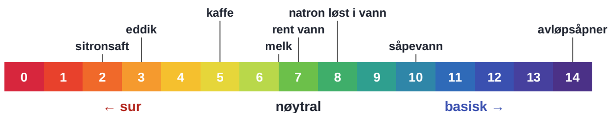
Figur 5.15 pH i noen vanlige produkter. Verdiene er omtrentlige.
