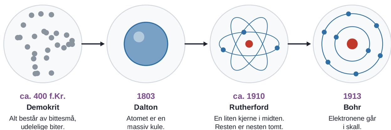
Figur 3.15 Atommodellen gjennom tiden.
