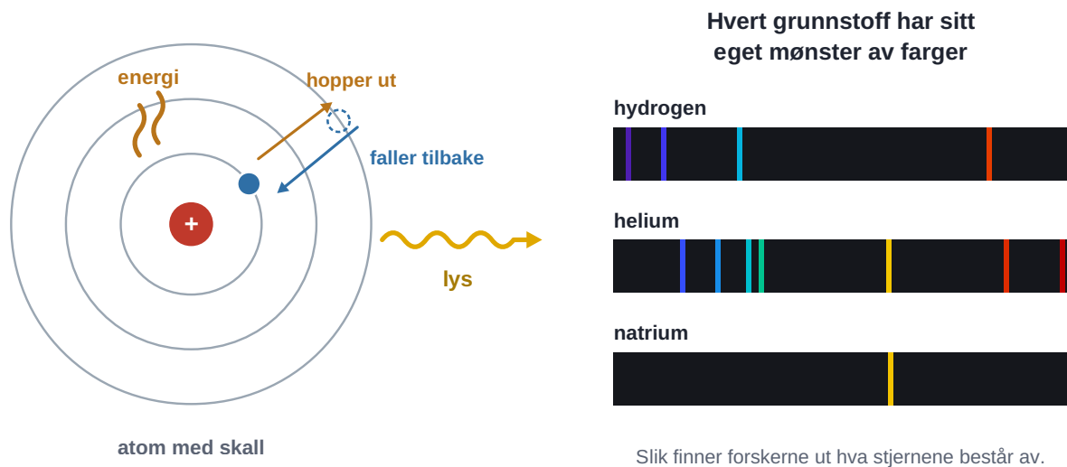
Figur 3.16 Elektronet hopper ut og faller tilbake og sender ut lys. Hvert grunnstoff har sitt eget mønster av farger.
