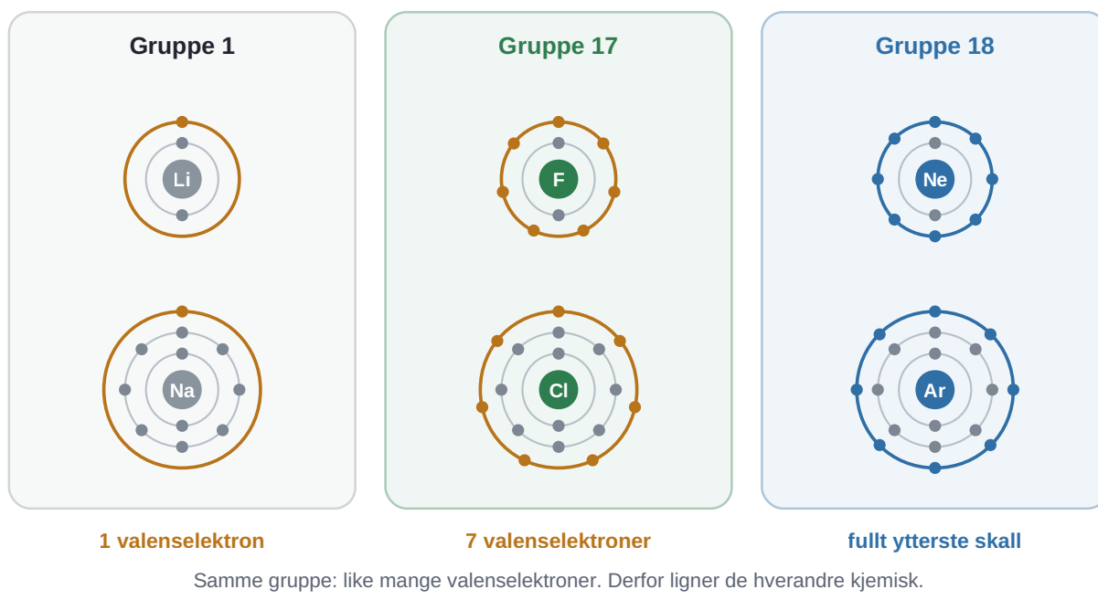
Figur 5.31 Grunnstoffene i samme gruppe har like mange valenselektroner.
