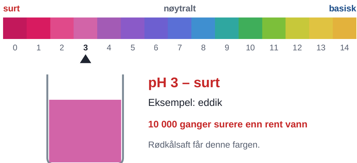
Figur 5.16 Prøv selv: pH-skalaen. På nettsiden kan du endre pH-verdien.
