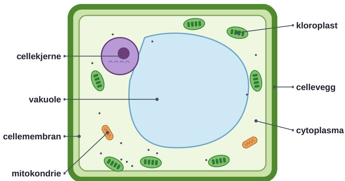
Figur 2.3 En plantecelle.
