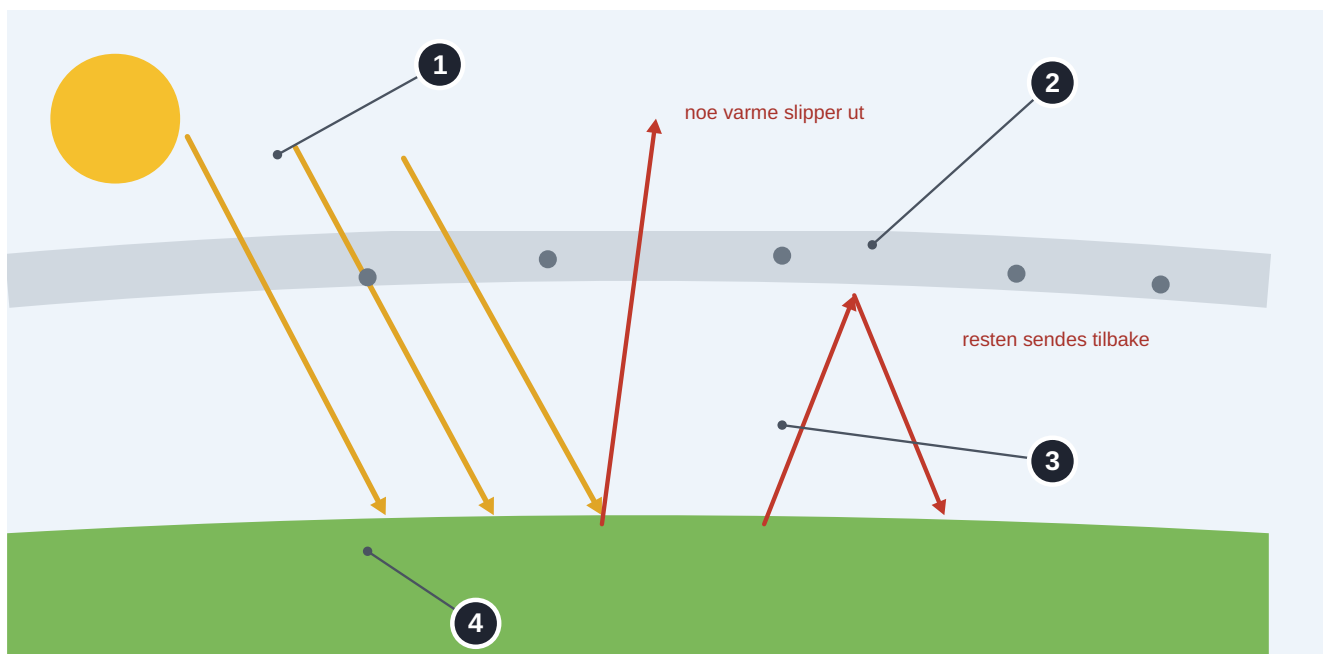
Figur 7.18 Drivhuseffekten til oppgavene.
