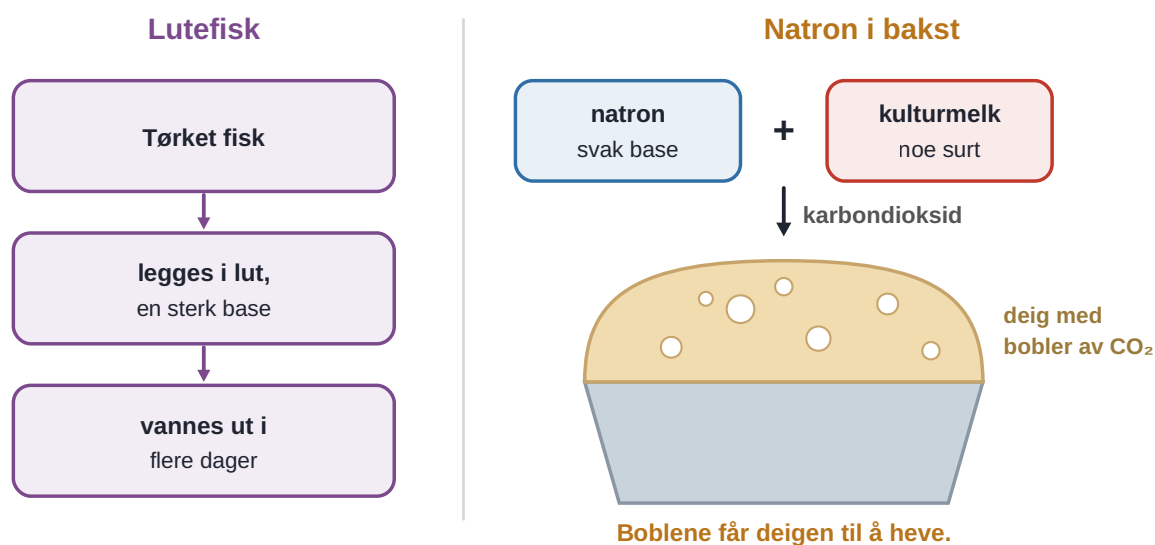
Figur 5.27 Baser i maten: lutfisk og natron i bakst.
