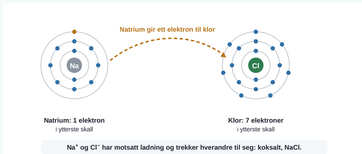
Figur 5.29 Ionebinding mellom natrium og klor.
