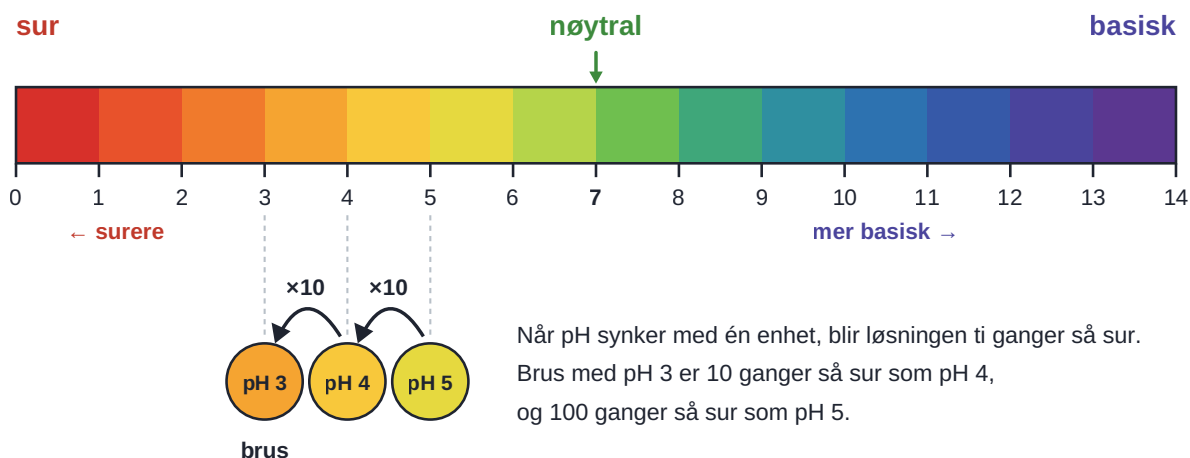
Figur 5.26 pH-skalaen. Når pH synker med én enhet, blir løsningen ti ganger så sur.
