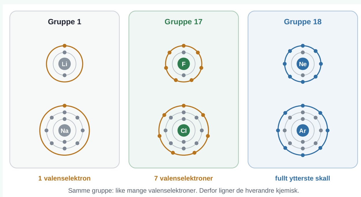
Figur 5.28 Grunnstoffene i samme gruppe har like mange valenselektroner.
