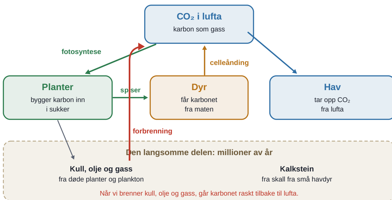
Figur 5.24 Karbonets kretsløp.
