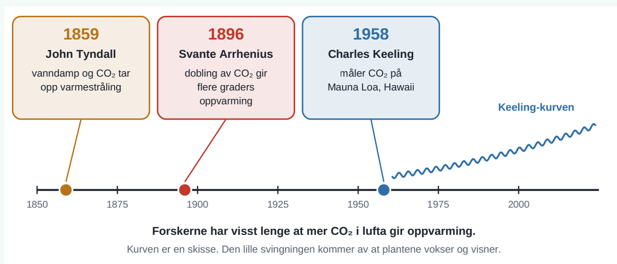
Figur 7.29 Kunnskapen om drivhuseffekten fra 1859 til i dag.
