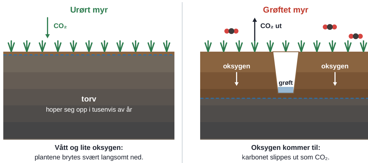
Figur 5.23 Urørt myr lagrer karbon. Grøftet myr slipper karbonet ut som \text{CO}_2 .
