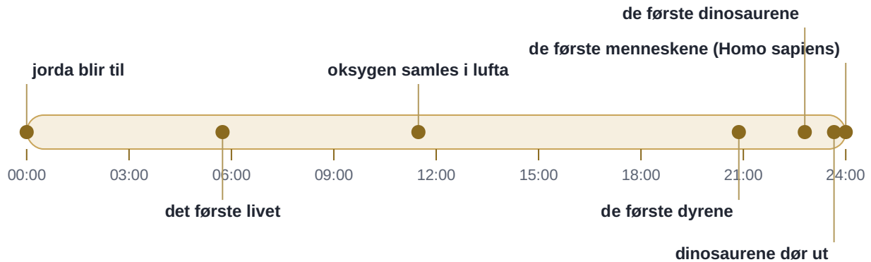
Figur 4.11 Hvis jordas historie var ett døgn, kom menneskene noen sekunder før midnatt.
