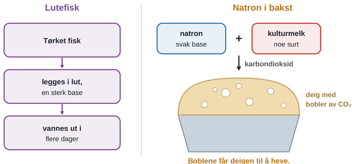
Figur 5.25 Baser i maten: lutefisk og natron i bakst.
