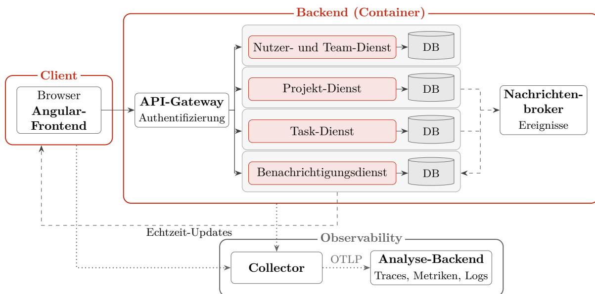
Abbildung 1: Geplante Architektur des Projektmanagement-Werkzeugs (vereinfacht). Durchgezogene Pfeile zeigen synchrone Aufrufe, gestrichelte Pfeile Ereignisse und gepunktete Pfeile Telemetriedaten.
