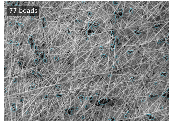
U-Net + CC
