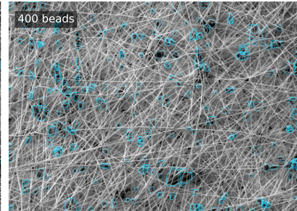
YOLOv8
