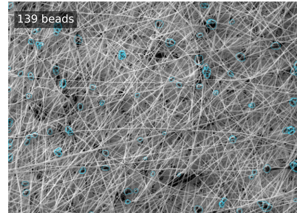
Mask R-CNN
