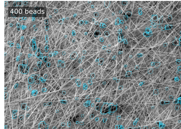
YOLOv8
