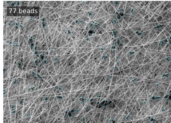
U-Net + CC
