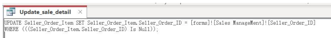
Figure32: Update_sale_detail SQL
