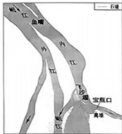
图 21 都江堰示意图
