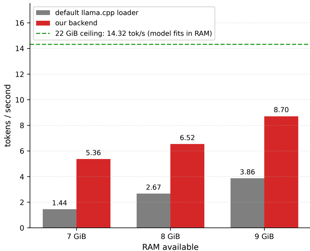
GPT-OSS-20B (12.85 GiB on disk)
