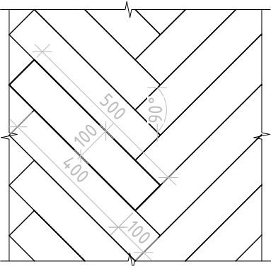
Рисунок паркета "ёлочка". М 1:15
