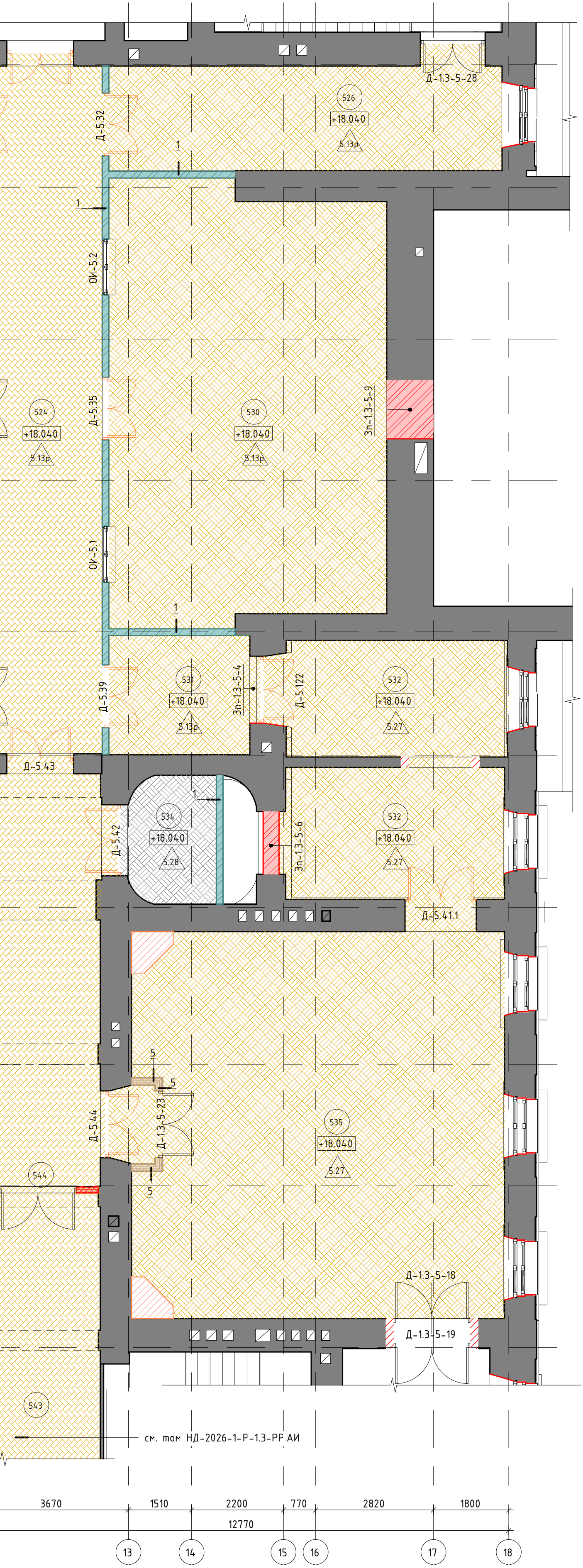
Маркировочный план фрагмента 5 этажа в осях 12-18/Д-Р
