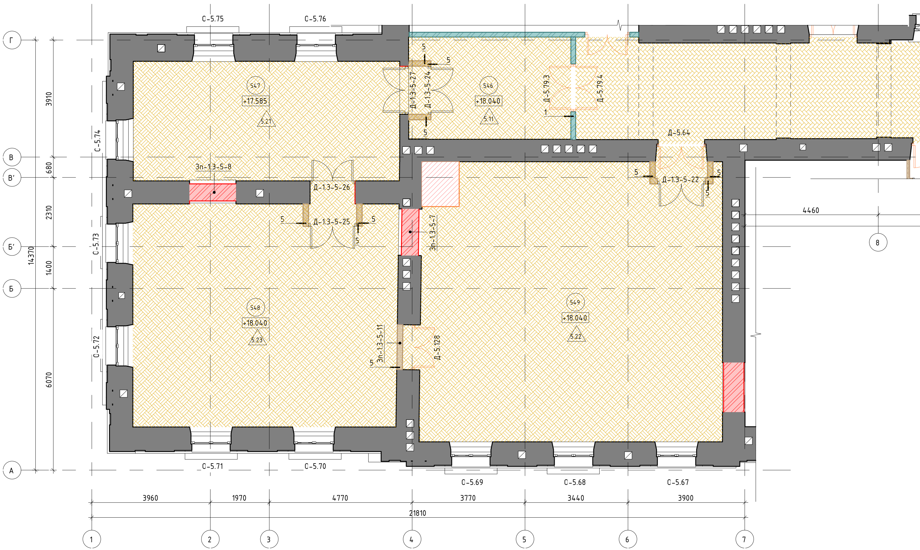
Маркировочный план фрагмента 5 этажа в осях 1-13/А-Г (1 : 75)
