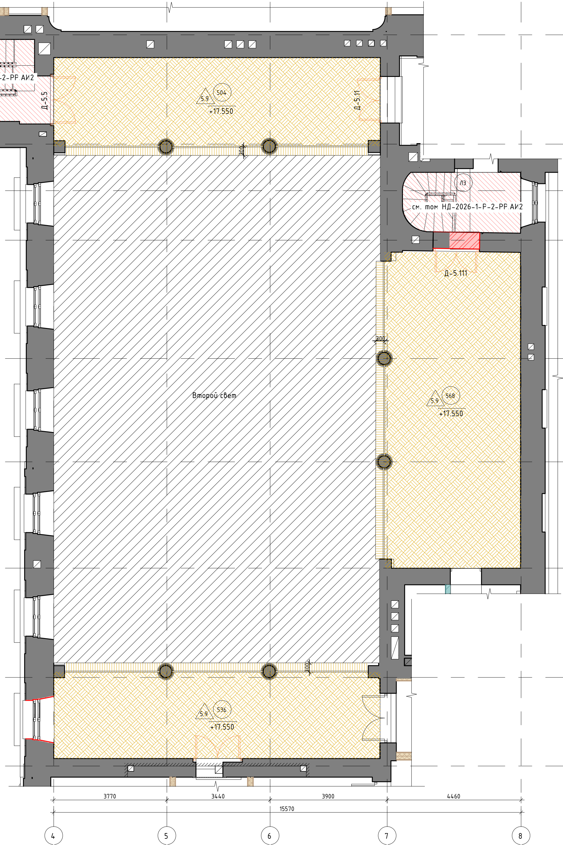
Маркировочный план фрагмента 5 этажа в осях 4–7/П–З
