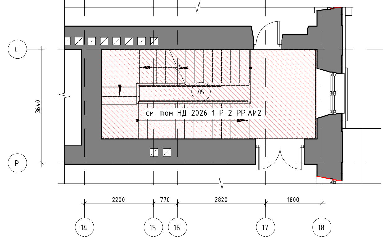
Маркировочный план фрагмента 5 этажа в осях 14–18/Р–С
