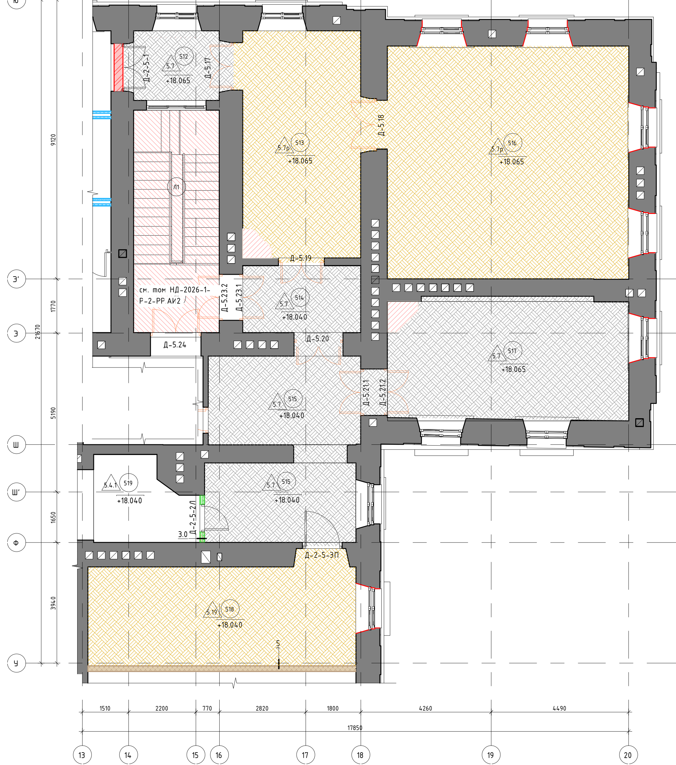
Маркировочный план фрагмента 5 этажа в осях 13-20/У–Ю
