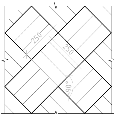
Рисунок паркета “корзинка”. М 1:15
