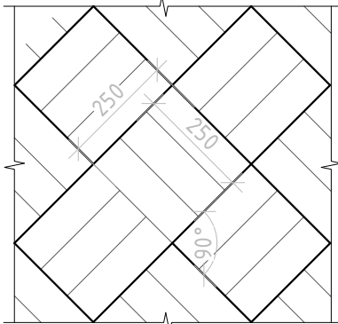
Рисунок паркета “корзинка”. М 1:15
