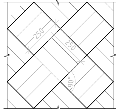
Рисунок паркета “корзинка”. М 1:15
