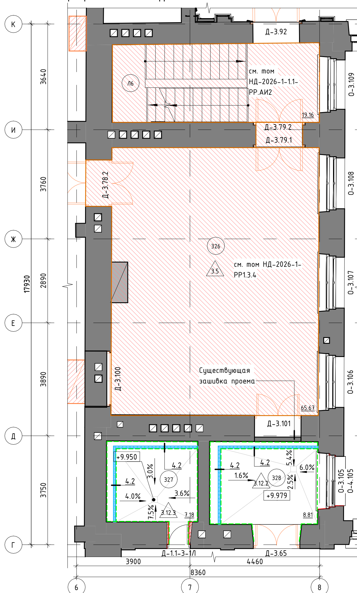
Маркировочный план фрагмента 3 этажа в осях 6-8/Г-К (1: 75)
