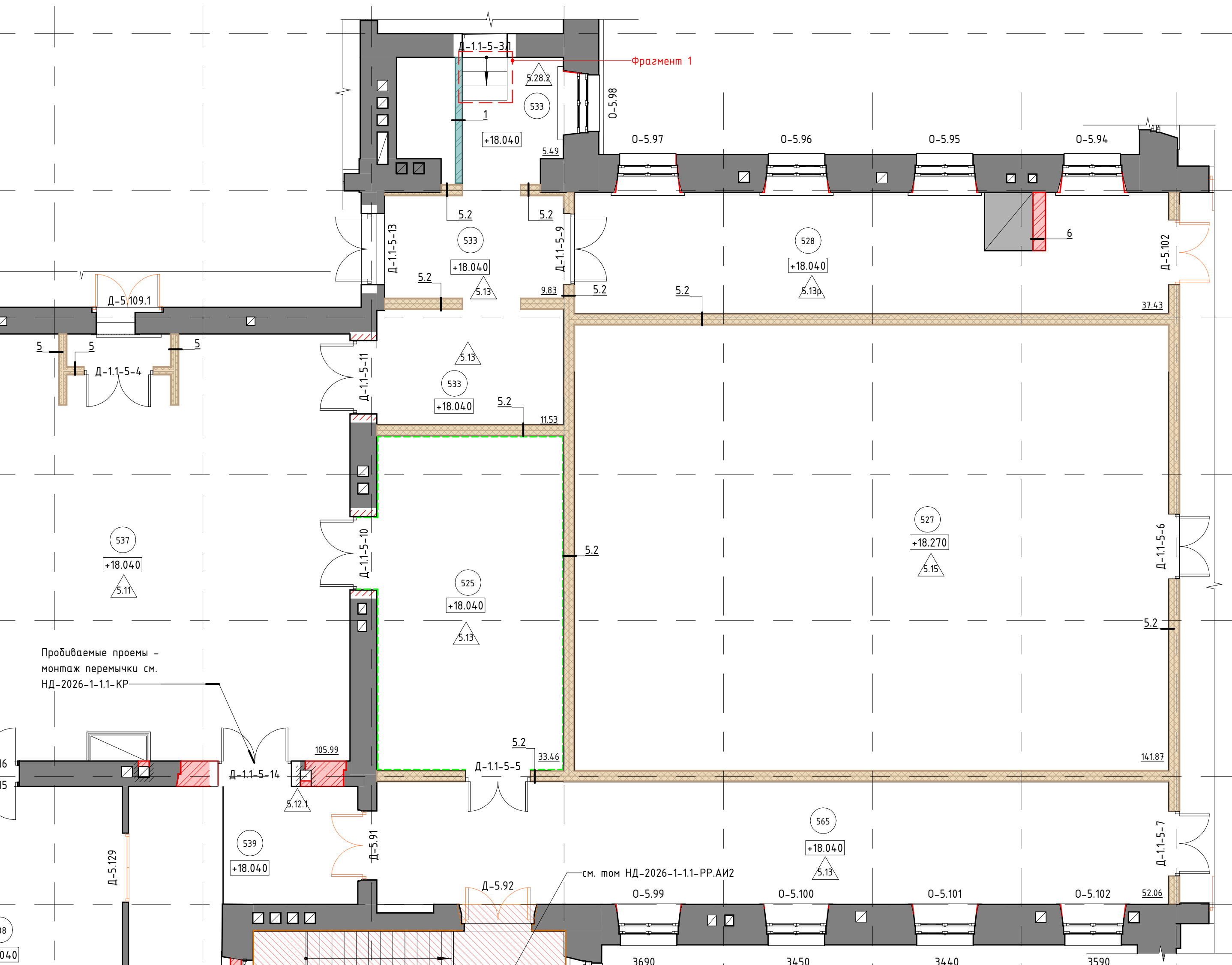
Маркировочный план фрагмента 5 этажа в осях 4-12/Г-С (1 : 75)
