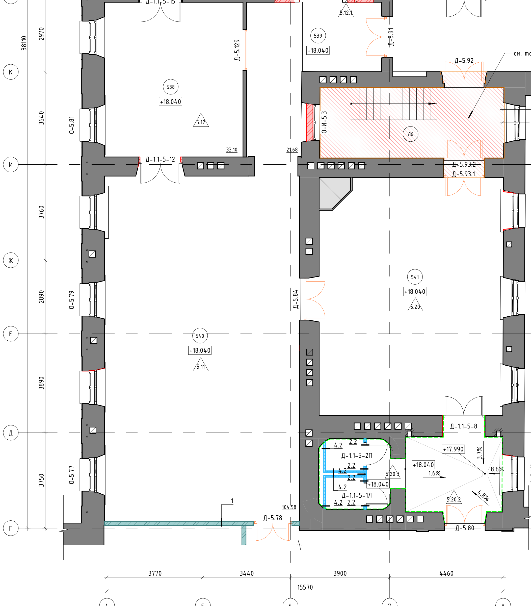
Экспликация помещений фрагмента 5 этажа в осях 4-12/Г-С
