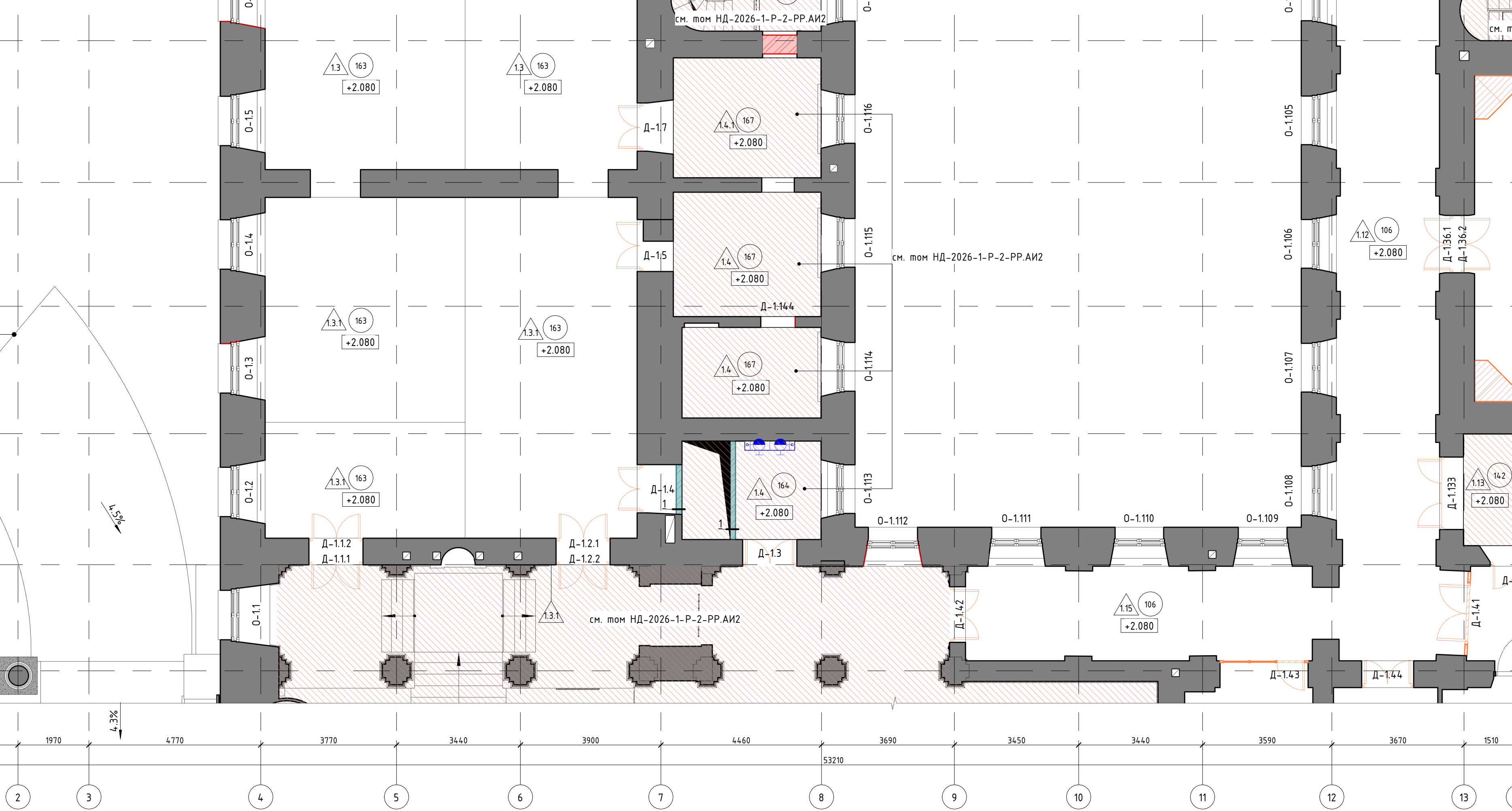
перегородок и стен по 1-20/П-Ю 1 этажа
