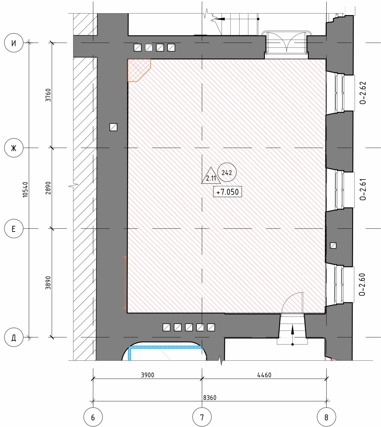
Маркировочный план фрагмента 2 этажа в осях 6-8/Д-И
