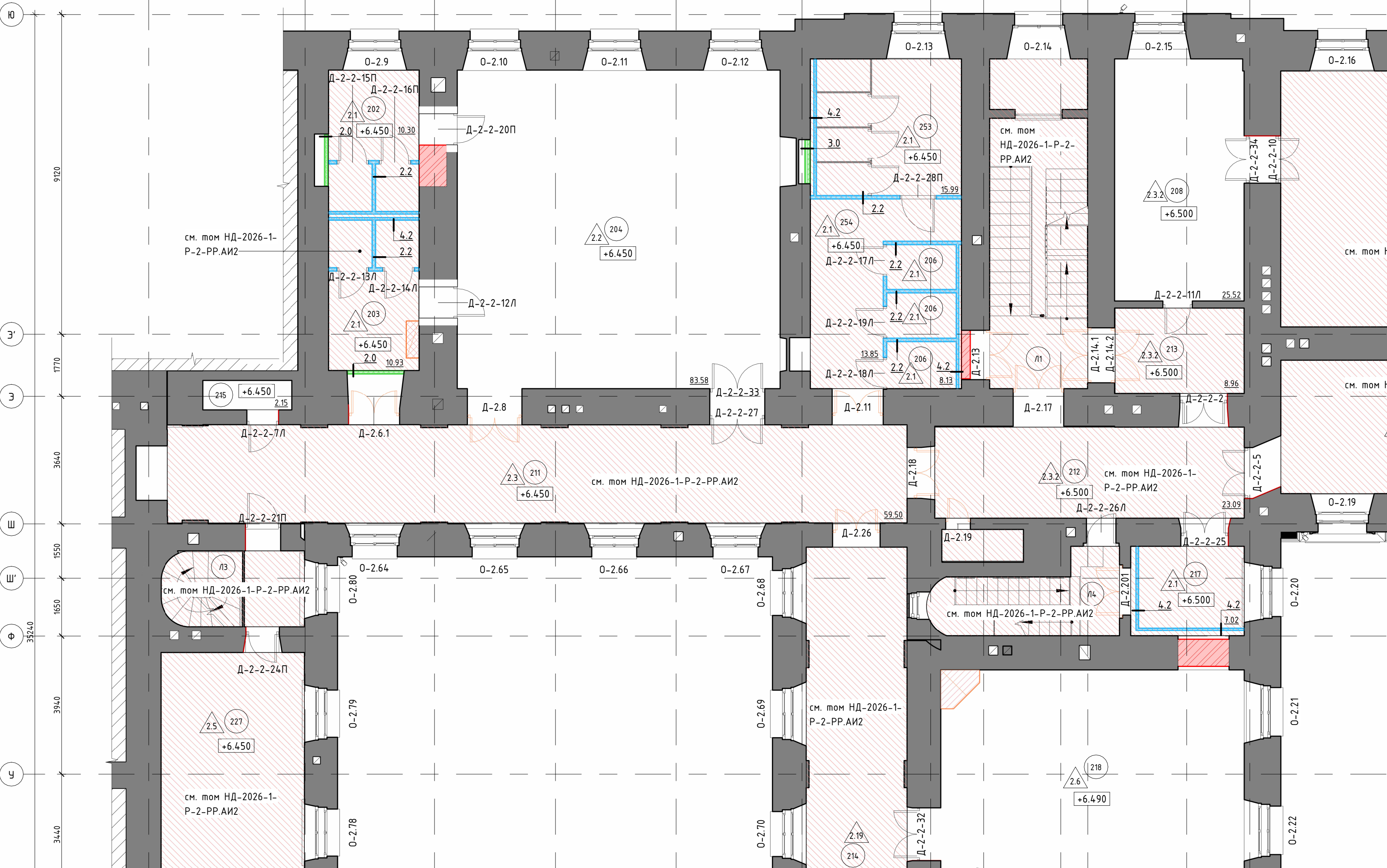
Маркировочный план фрагмента 2 этажа в осях 7-20/П-Ю
