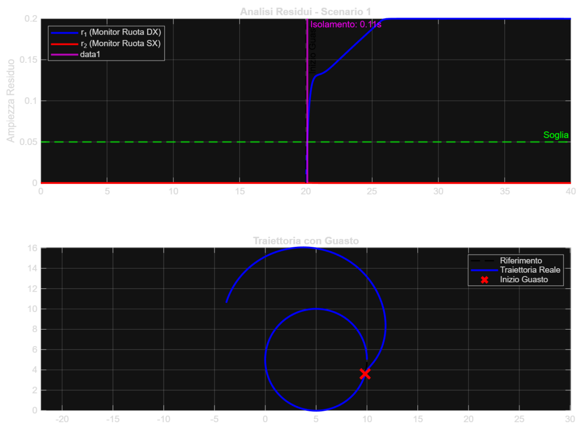
Figura 4.1: Isolamento del guasto nello Scenario 1 (FD1): Il residuo r_1 isola il guasto sulla ruota destra in 0.110s mentre r_2 rimane nullo.
