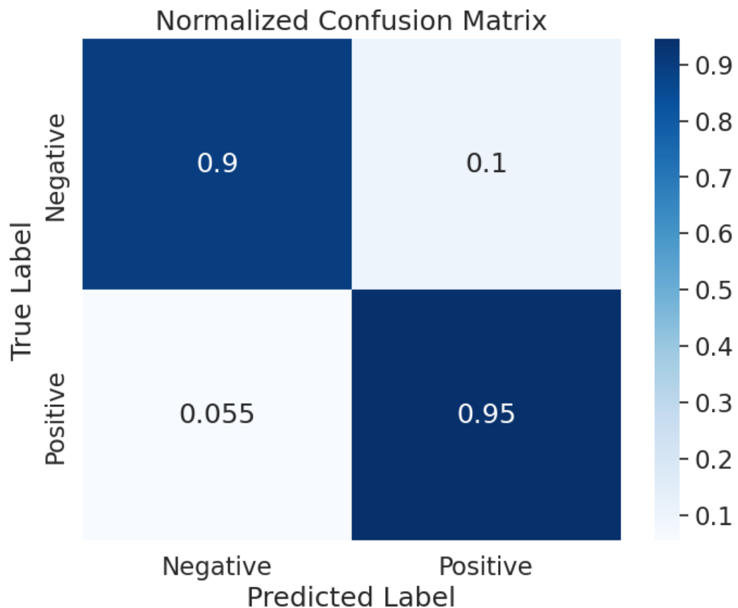
Figura 4.1: Matrice di confusione
