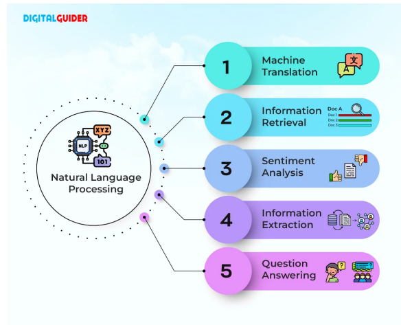
Figura 1.1: Funzionamento NLP
