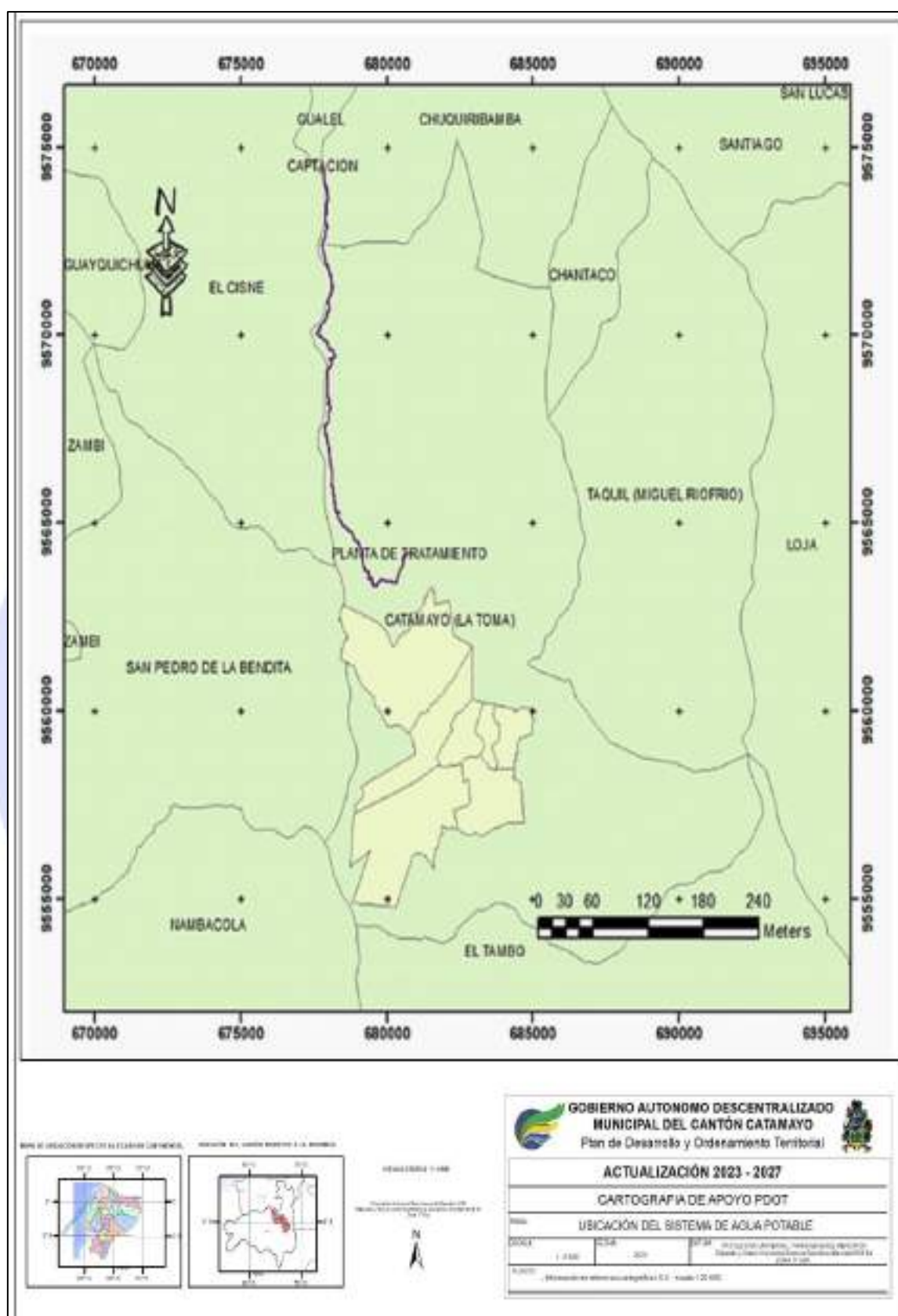
Mapa 37. Ubicación del sistema de agua potable de la ciudad de Catamayo
