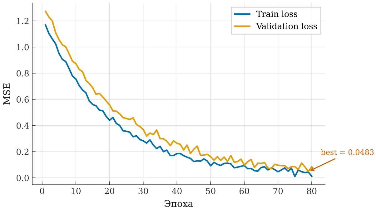
Сходимость обучения MLP-FNO модели
