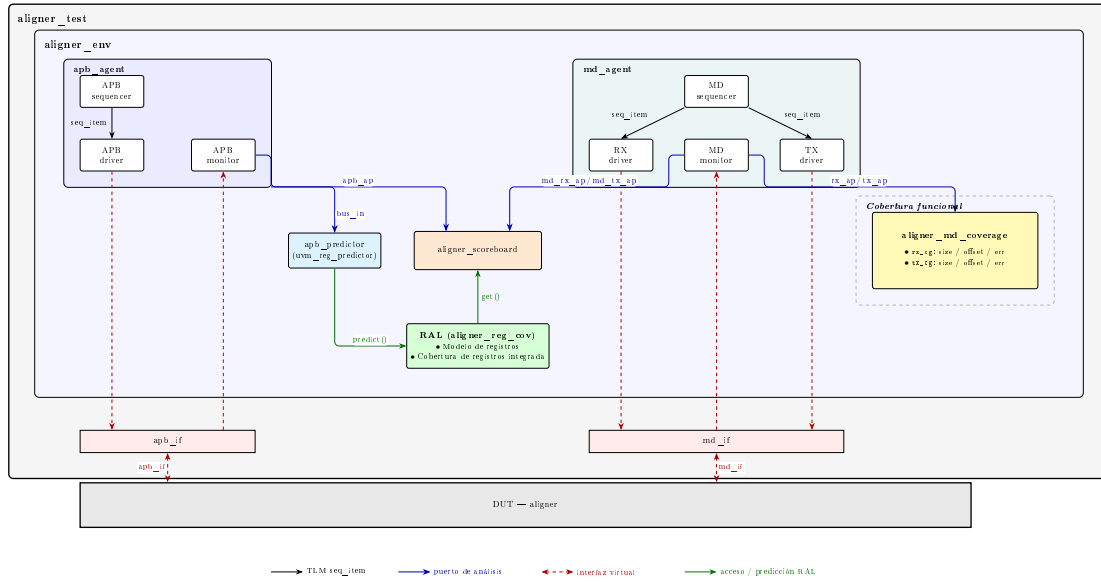
Figura 1. Arquitectura del ambiente de verificación UVM. Los drivers conducen el DUT a través de las interfaces virtuales; los monitors publican las transacciones observadas hacia el scoreboard por puertos de análisis. El RAL se conecta al secuenciador APB mediante el adaptador y se sincroniza con el scoreboard por medio del predictor y get() .
