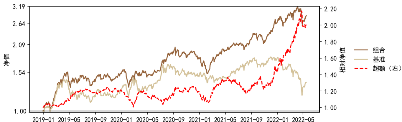
图 4：小市值 400、低波动、低价股、小市值 100 四因子增强策略
