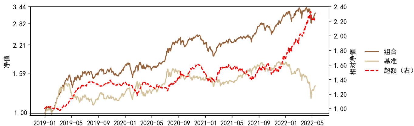
图 5：小市值、低波动、高贝塔、高利润增长四因子增强策略
