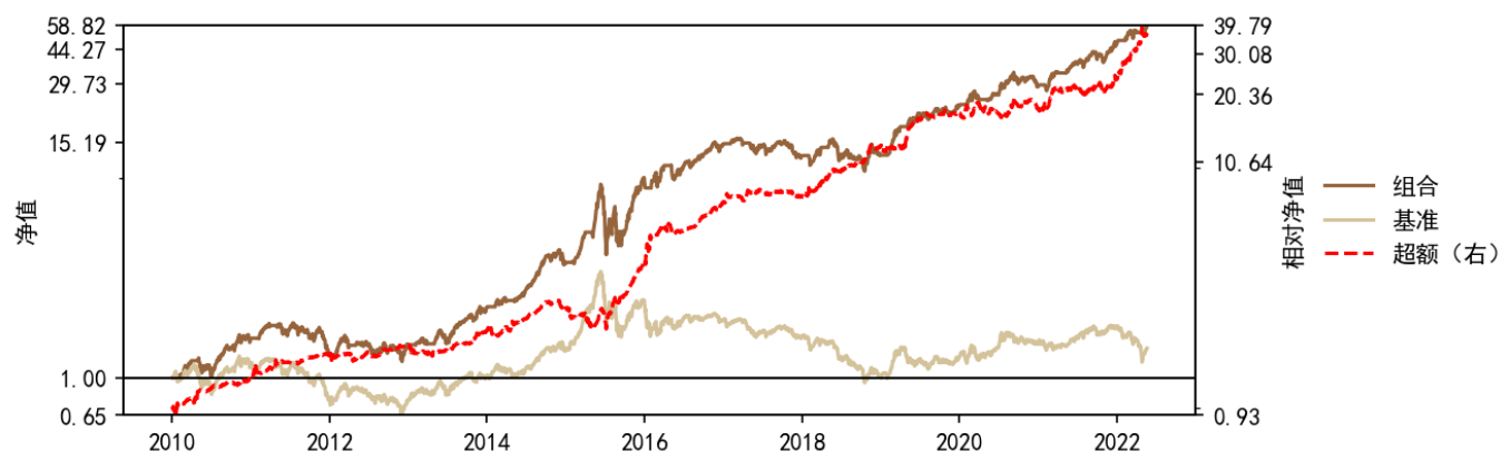
图 12：择时小市值 100 策略回测结果
