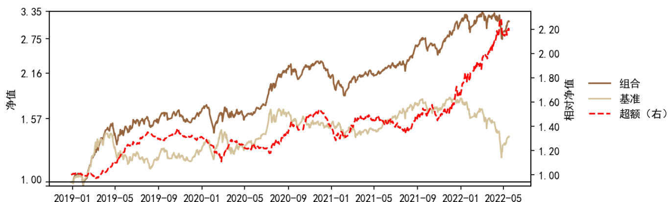
图 9：小市值、低波动、高贝塔、小市值、高季度净资产回报率五因子增强策略
