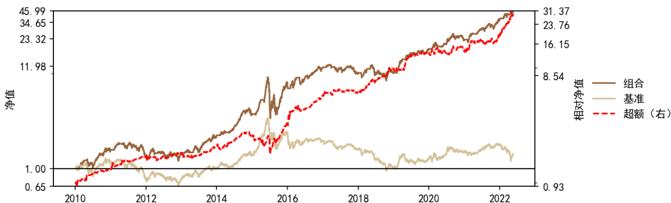
图 16：带跌停惩罚的择时小市值 100 回测结果
