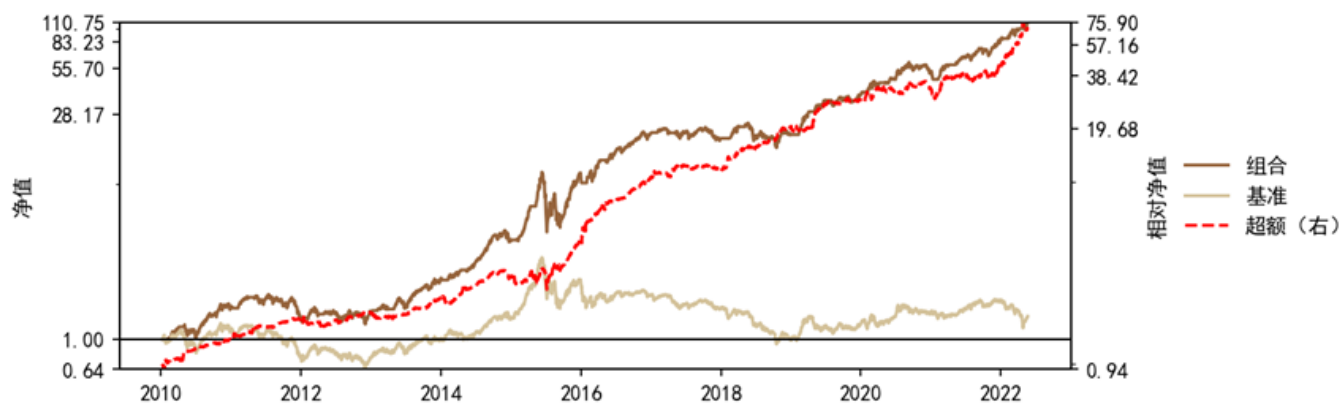
图 18：双周调仓和带跌停惩罚的择时小市值 100 策略回测结果
