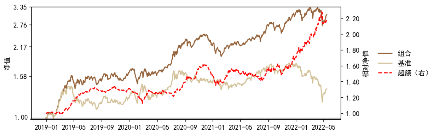
图 7：小市值、低波动、高贝塔、高利润增长、季度净资产回报率五因子增强策略
