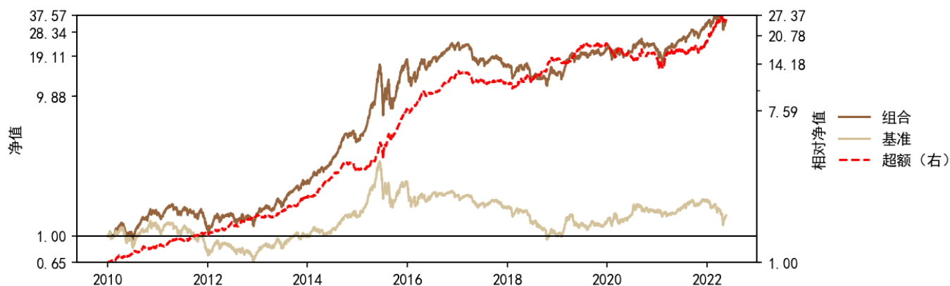
图 10：小市值 50 回测结果
