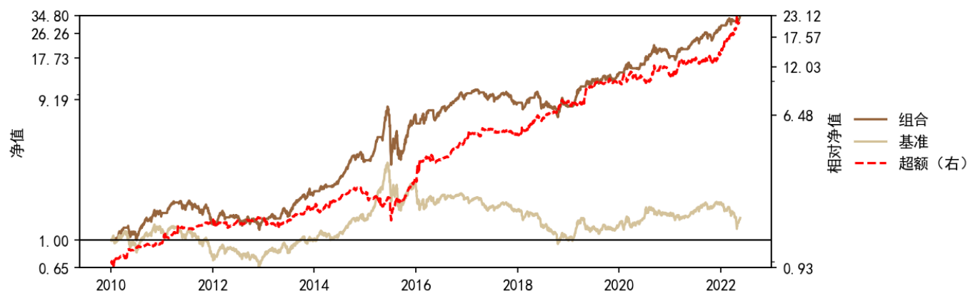
图 20：季度调仓和带跌停惩罚的择时小市值 100 策略回测结果
