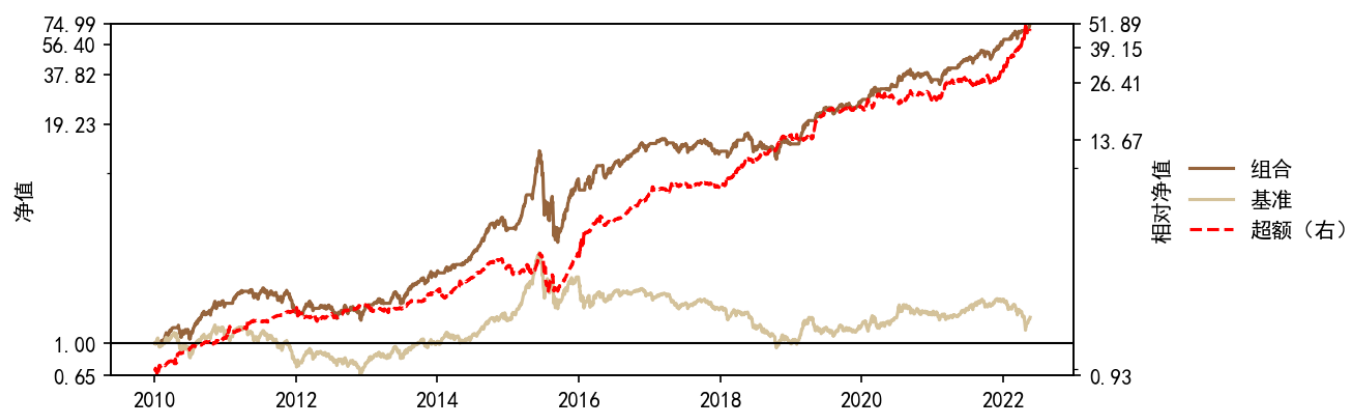
图 17：单周调仓、带跌停惩罚的择时小市值 100 策略的回测结果
