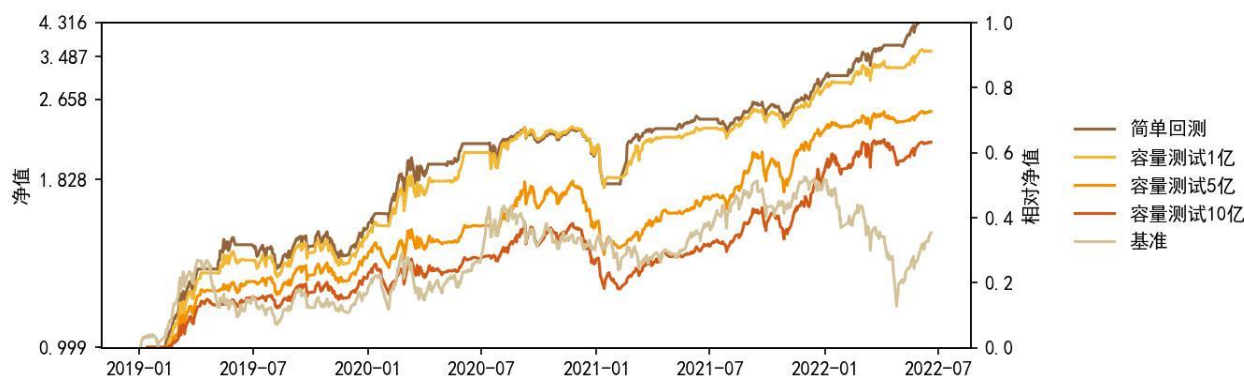
图 22：择时双周频小市值低波 100 策略（容量测试）
