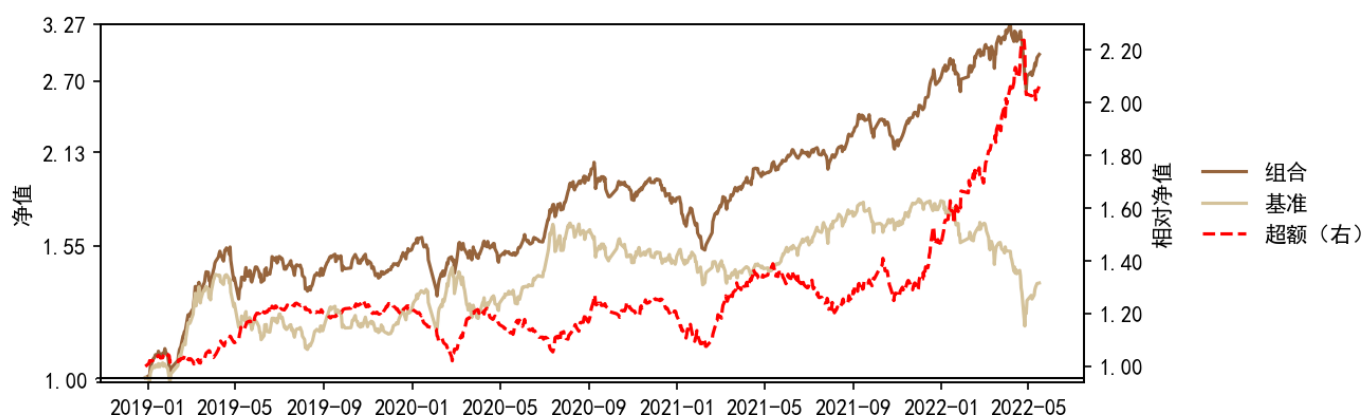
图 3：小市值、低波动、低价股三因子增强策略
