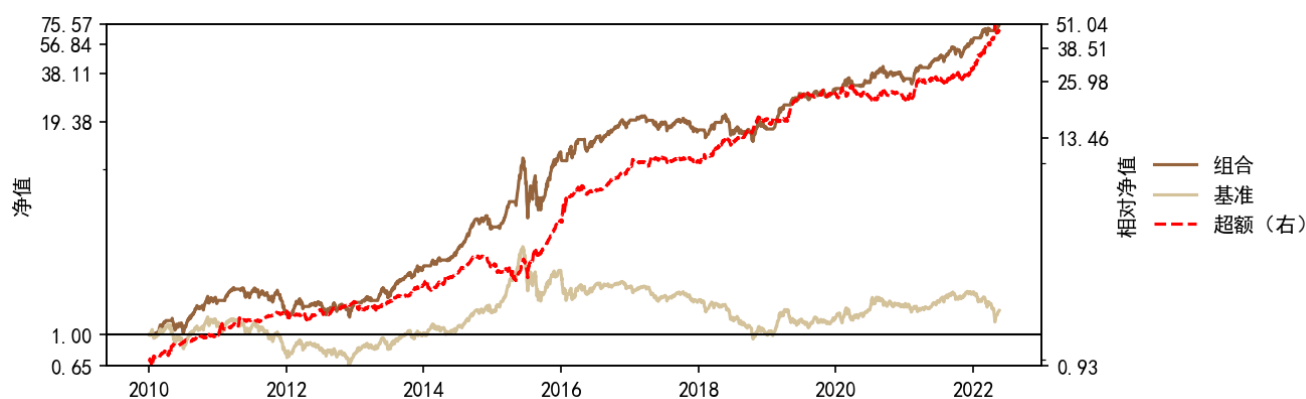
图 13：择时小市值 50 策略回测结果
