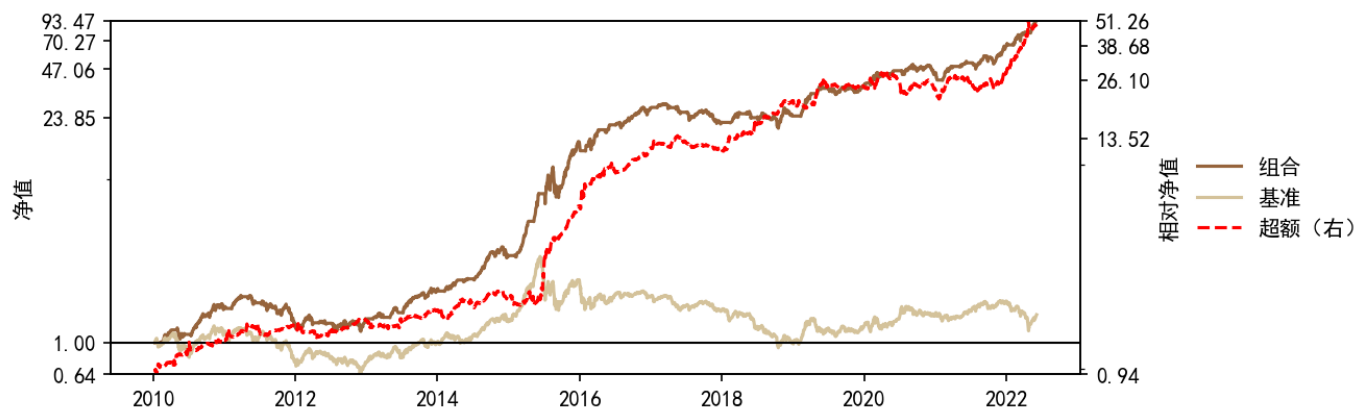
图 23：择时双周频小市值低波 100 策略（费用测试）
