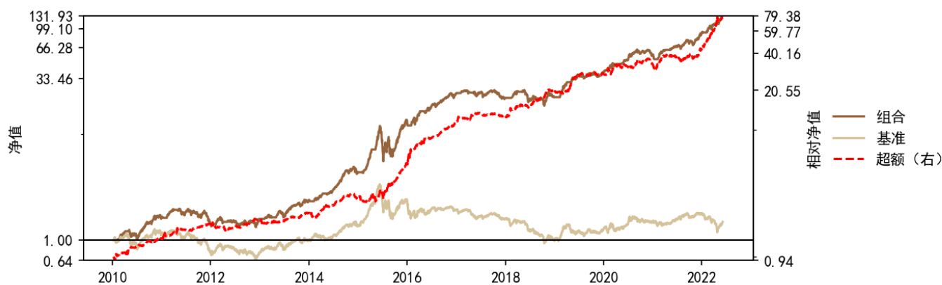
图 25：择时双周频小市值低波 50 策略（保留六月持仓）
