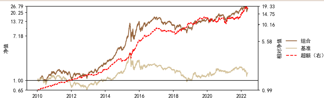
图 1：小市值 100 策略回测结果
