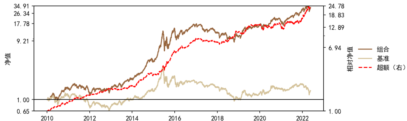
图 11：小市值低波 50 策略回测结果
