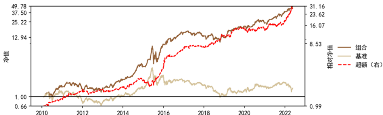
图 15：月末调仓的择时小市值低波 50 策略回测结果
