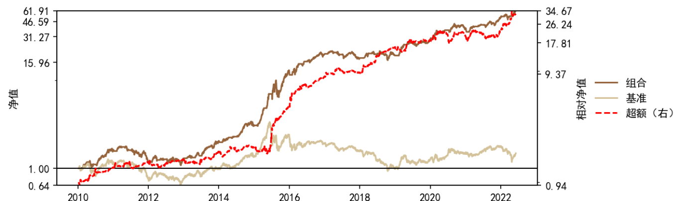
图 24：择时双周频小市值低波 50 策略（分析师覆盖测试）
