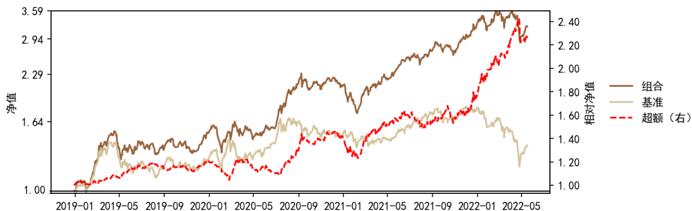
图 8：非流动性、小市值、高增长、低动量、高波动五因子增强策略
