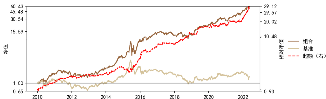
图 14：择时小市值低波 50 策略回测结果
