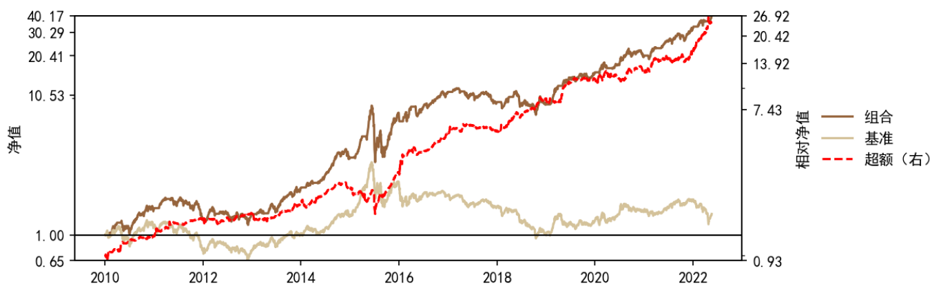
图 19：双月调仓和带跌停惩罚的择时小市值 100 策略的回测结果
