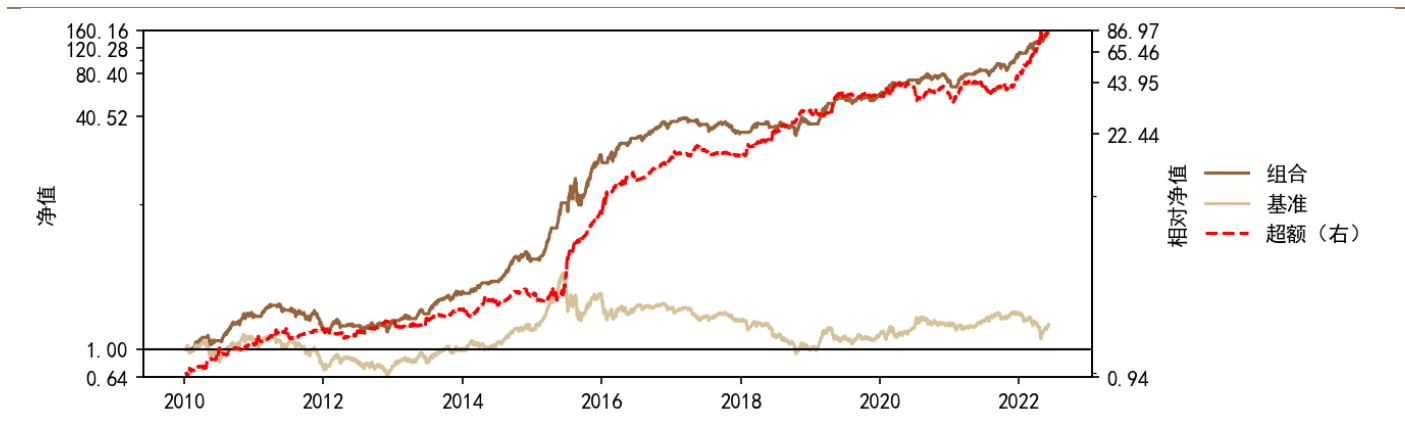
图 21：择时双周频小市值低波 50 策略
