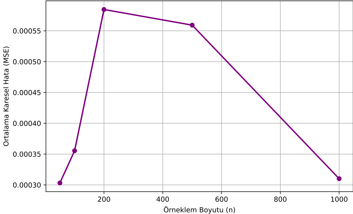
Örneklem Boyutunun MSE Üzerindeki Etkisi
