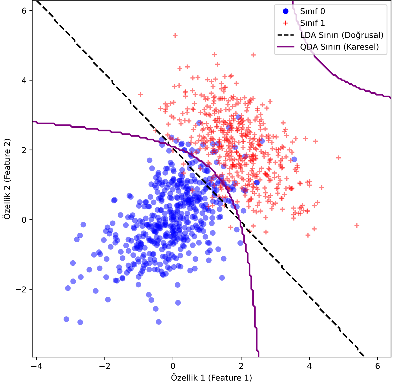
Eğitim Kümesi ve Karar Sınırları ( a=2 , \rho=0.5 )
