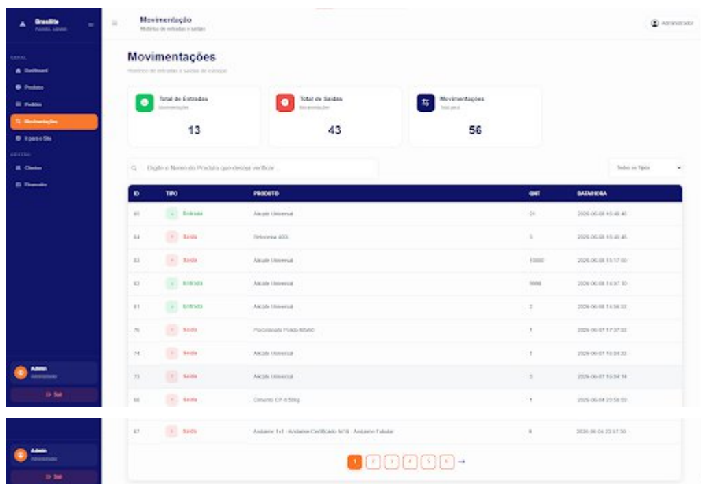
Figura 28 - Interface da seção de histórico e gerenciamento de movimentações de estoque no painel administrativo
