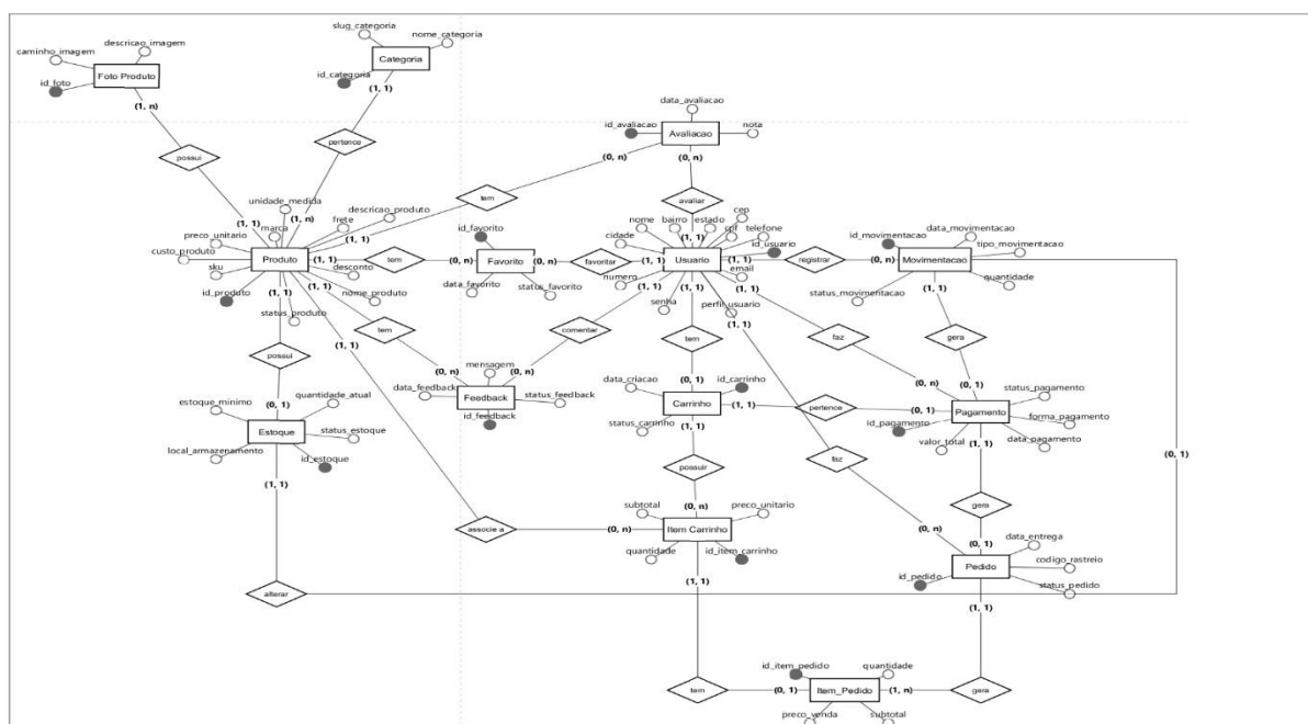
Figura 3 - Modelo conceitual do banco de dados do sistema
