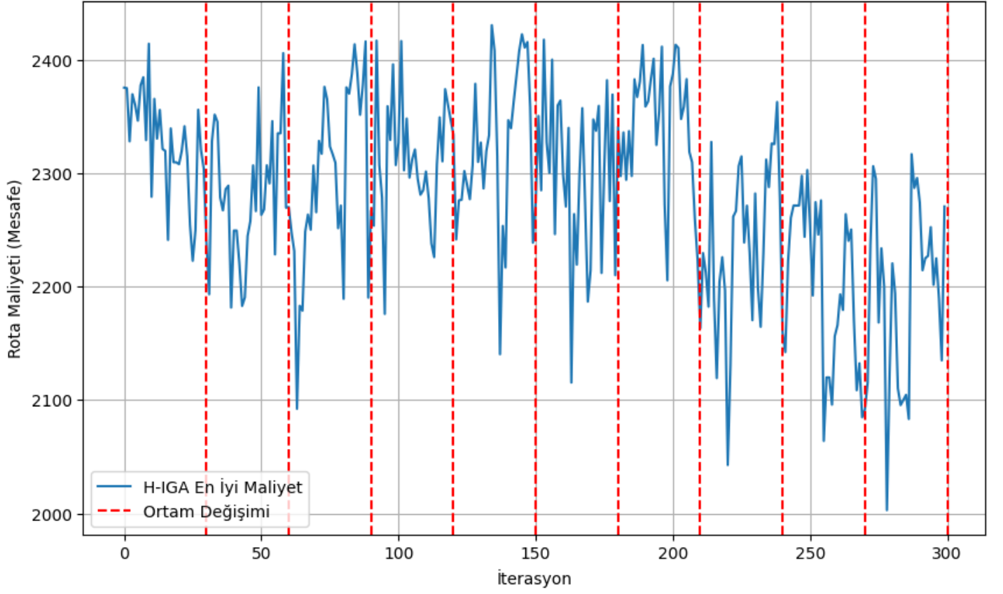
Dinamik TSP: H-IGA Performansı
