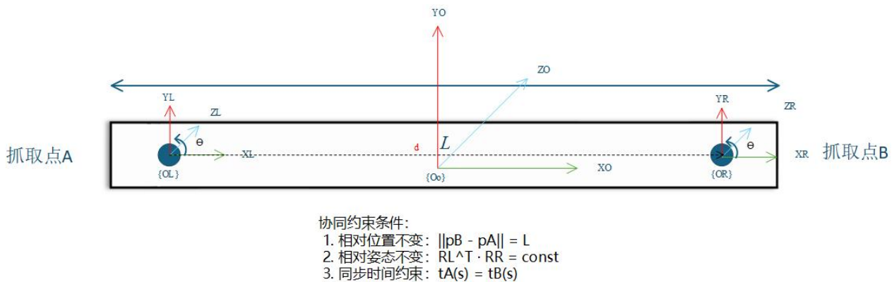
图 5 协同约束建模示意图
