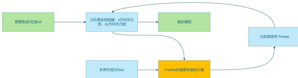
图 4 力位混合控制原理示意图
