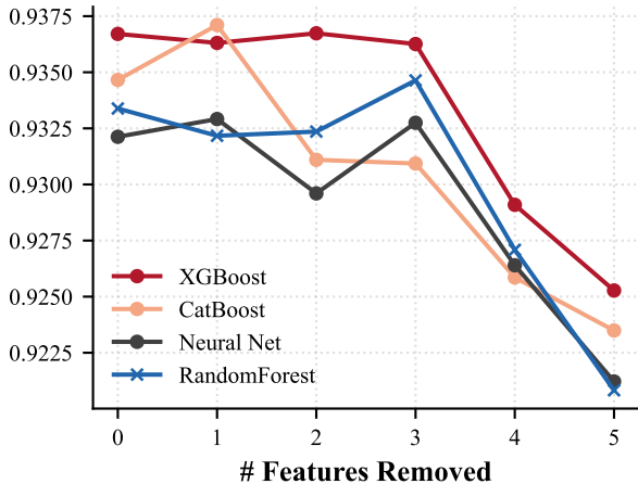
Test ROC-AUC
