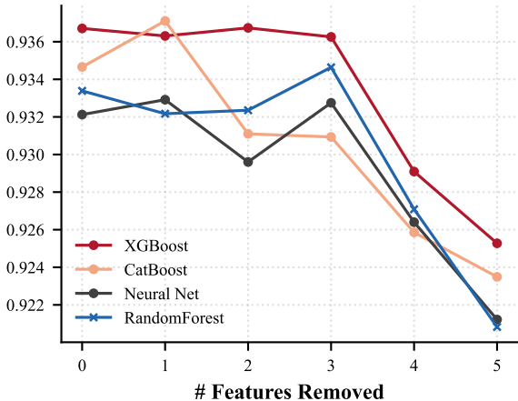
Test ROC-AUC
