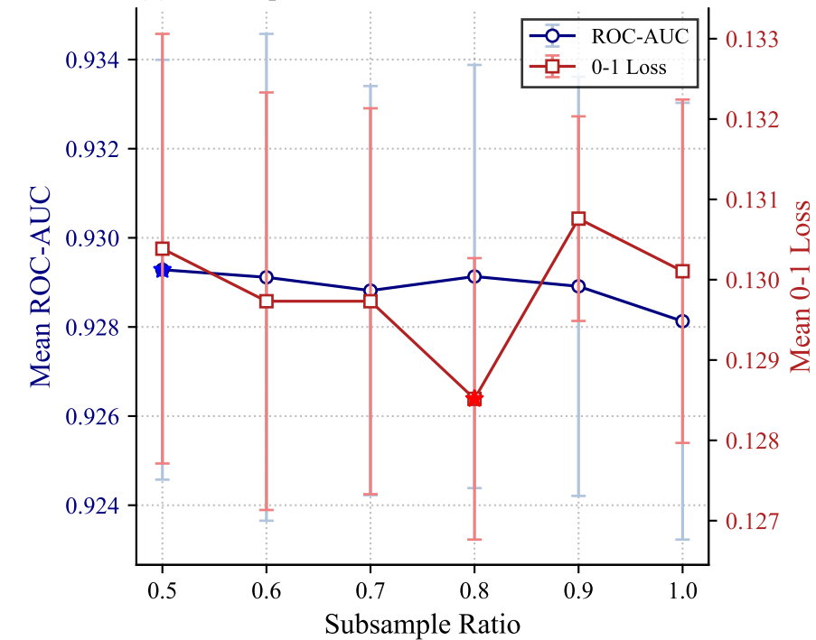
(d) Subsample Ratio
